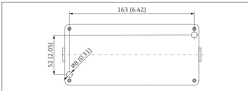
11 Gabarit de montage pour boîtier avec module électronique déporté. Unité de mesure mm (in)
