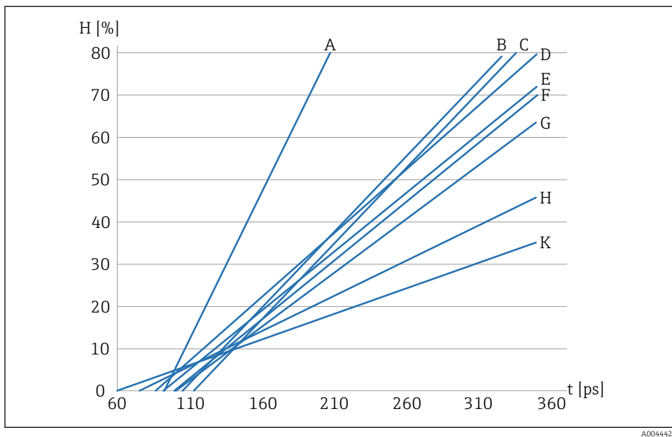
15 Ensemble de courbes d'étalonnage B (Cal.A, Cal.B, Cal.C, Cal.D, Cal.E, Cal.F, Cal.G, Cal.H, Cal.K)
