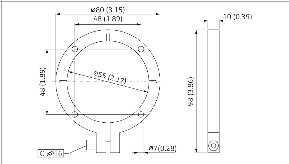
11 Brida de montaje para el sensor de varilla. Unidad de medida mm (in)
