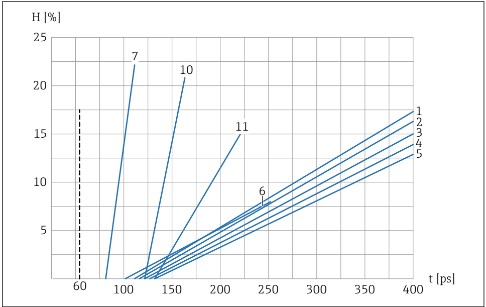
21 Conjunto de curvas de calibración A (Cal.1, Cal.2, Cal.3, Cal.4, Cal.5, Cal.6, Cal.7, Cal.10, Cal.11)
