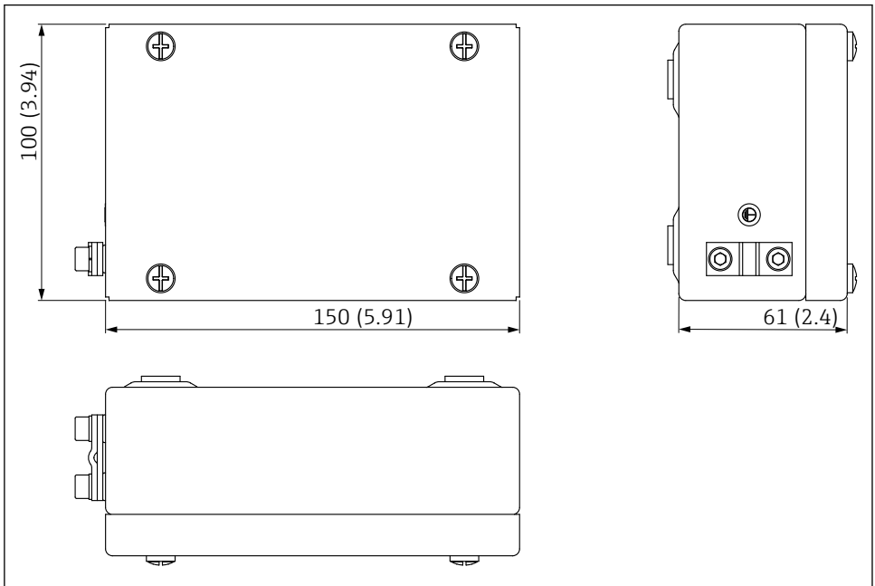
9 Medidas de la caja del sistema electrónico ATEX. Unidad de medida mm (in)
