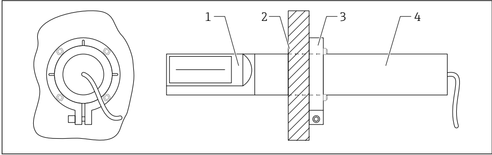
10 Sensor de varilla montado, vista posterior
