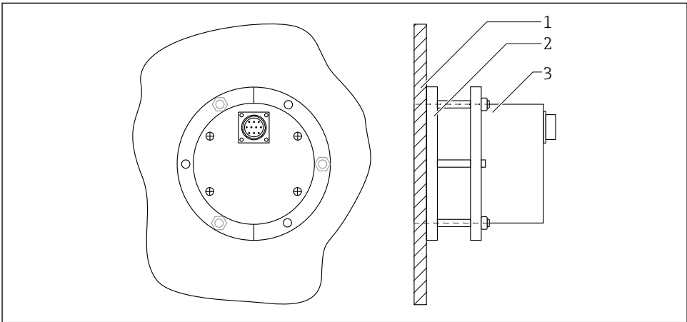
6 Sensor redondo montado, versión larga, vista posterior
