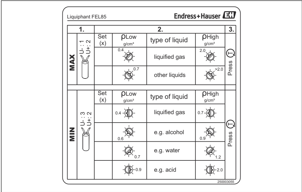
Resim: Sensör kartı
