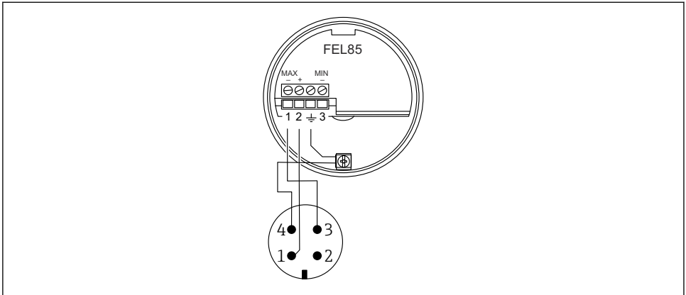
14 Klembezetting met M12-connector, MAX-bedrijfsmodus
