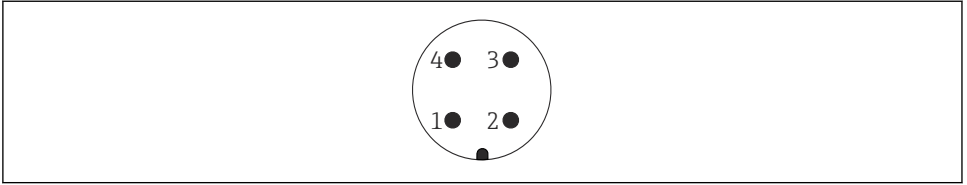
☞ 14 M12 플러그, 핀 할당
