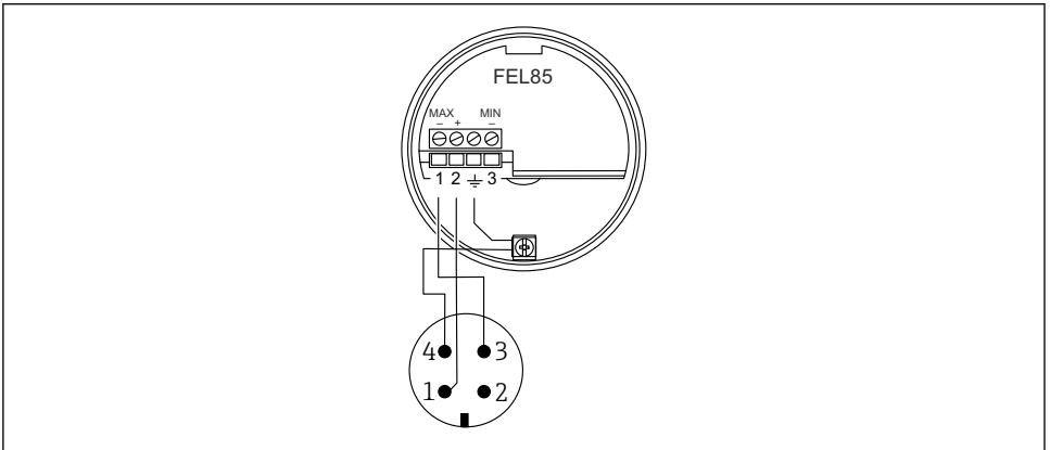
☞ 15 M12 커넥터의 단자 할당, MAX 작동 모드
