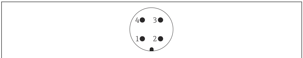
14 Fișa M12, alocarea pinilor
