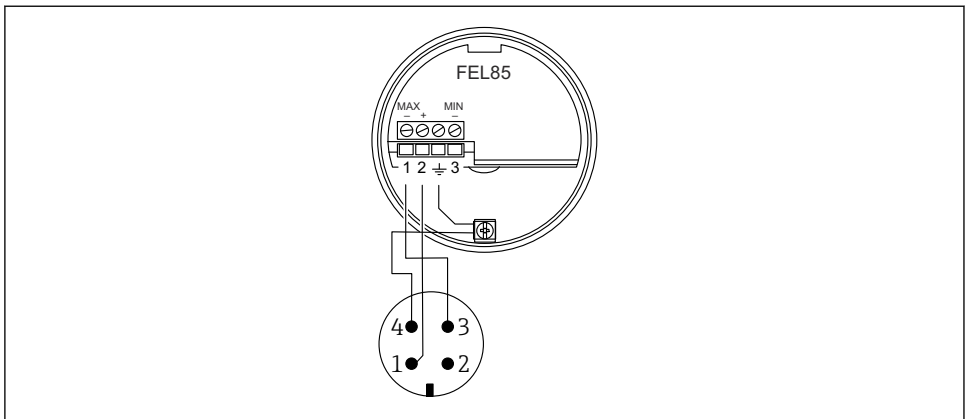
15 Alocarea bornelor cu conector M12, modul de operare MAX
