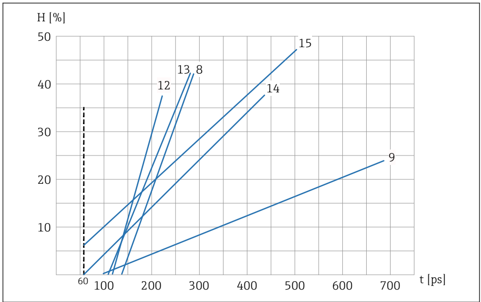
20 Curva de calibração definida como A (Cal.8, Cal.9, Cal.12, Cal.13, Cal.14, Cal.15)
