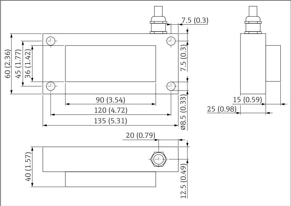
6 Dimensões. Unidade de medida mm (in)
