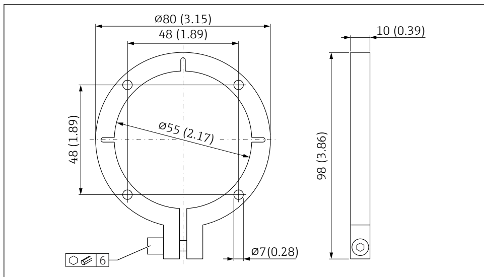
9 Flange de instalação para o sensor de haste. Unidade de medida mm (in)
