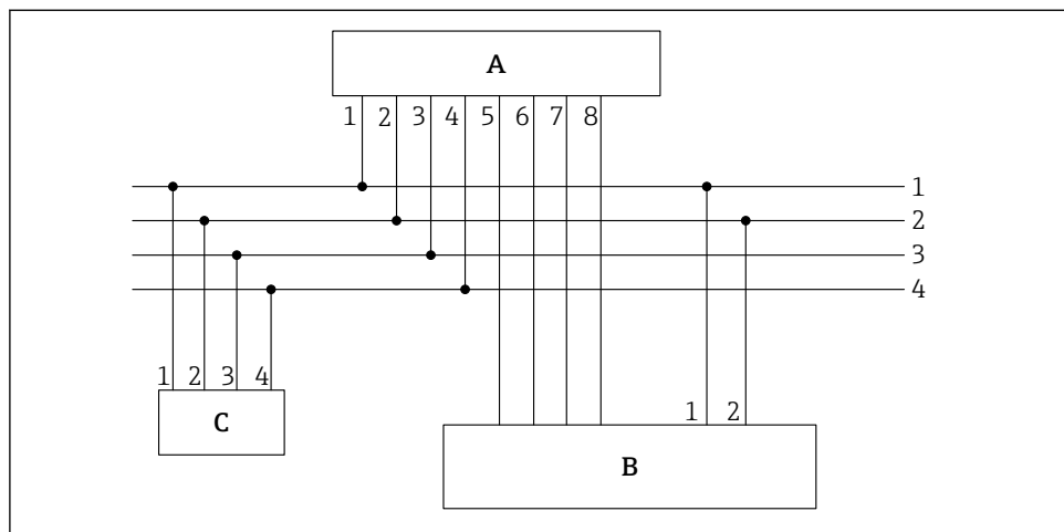
17 Exemplo de conexão, cabo com soquete de 10 pinos (no lado do equipamento) e arruelas na extremidade do cabo
