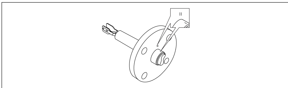
10 Lega merilnih vilic pri vodoravni namestitvi v posodo z uporabo oznake
