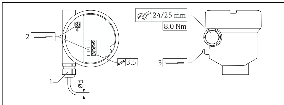
16 Primer spojke z vodom za kabel, elektronski vložek s priključnimi sponkami
