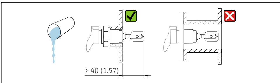
6 Příklad instalace pro vysoce viskózní kapaliny. Jedinota měření mm (in)
