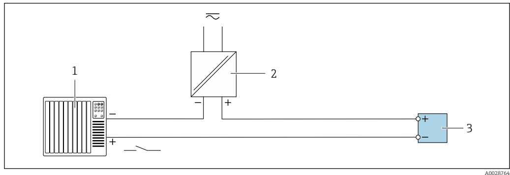
29 Exemplo de conexão para entrada de status
