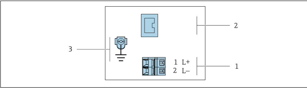
8 PROFINET 型仪表的接线端子分配
