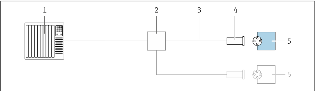
11 接线实例：PROFINET
