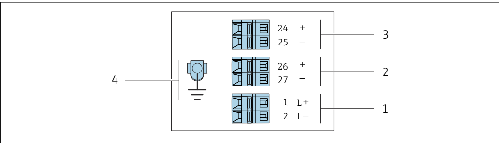
图 8 接线端子分配: 4...20 mA HART 或脉冲/频率/开关量输出
