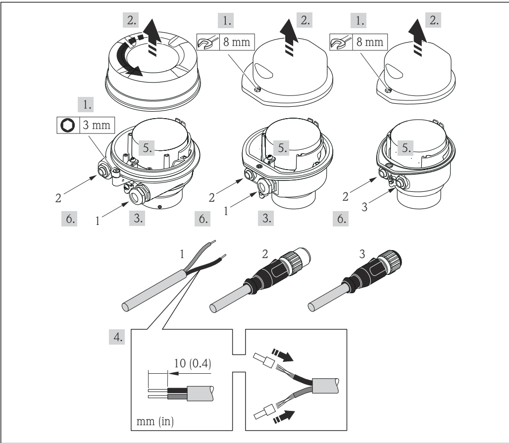
图 10 设备类型和连接实例
