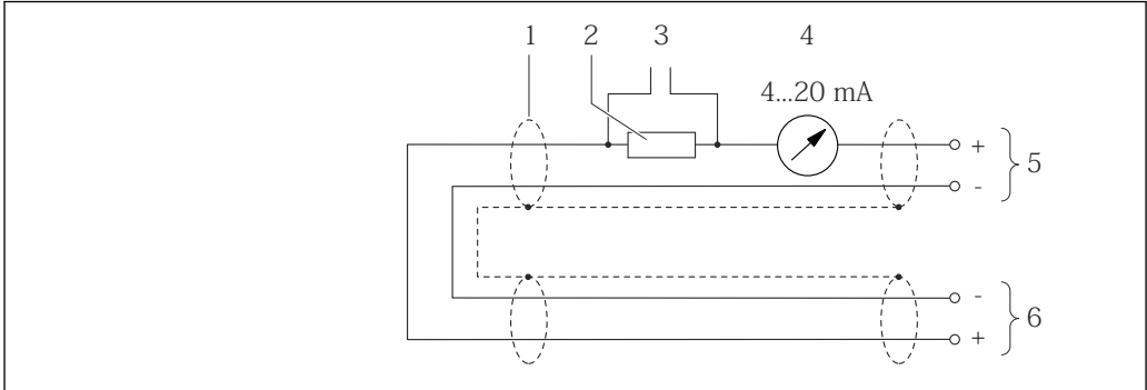
图 15 接线示例: HART 电流输入 (burst 模式), HART 电流输出 (有源信号)
