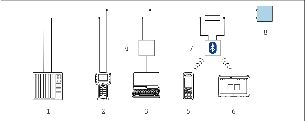
图 18 通过 HART 通信实现远程操作
