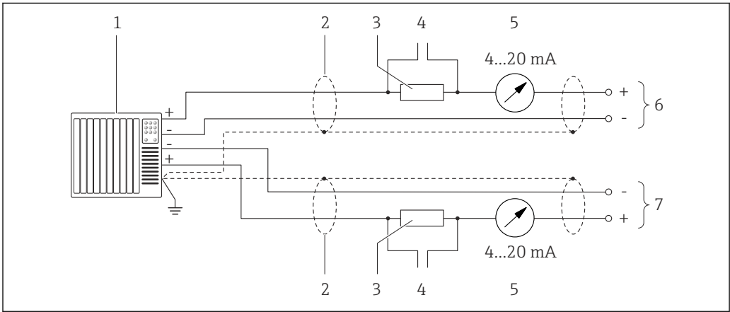
图 16 接线示例: HART 电流输入 (主站模式), HART 电流输出 (有源信号)
