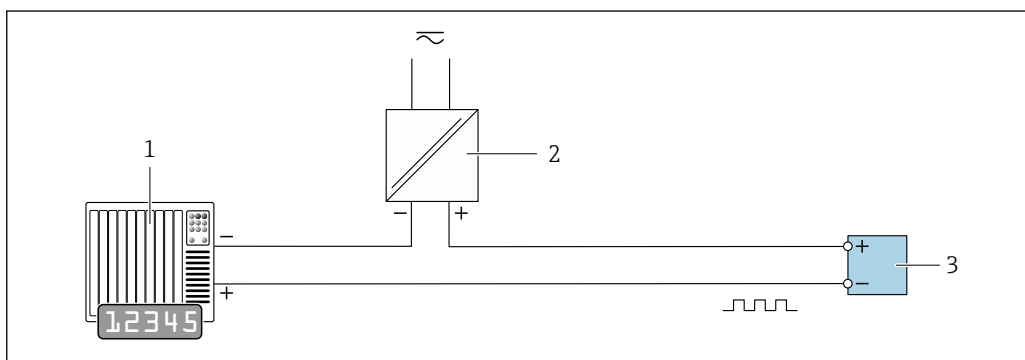
图 13 接线实例：脉冲/频率输出（无源信号）
