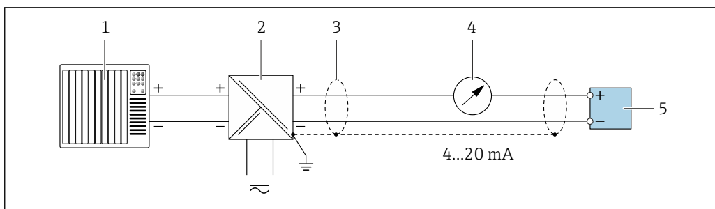
图 12 接线实例：4...20 mA HART 电流输出（无源信号）
