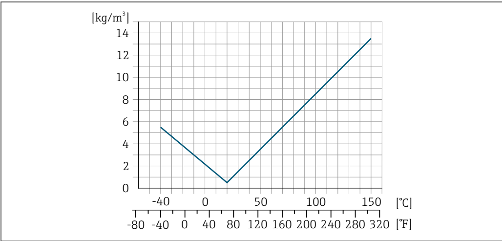
图 20 现场密度校正，例如在+20 °C (+68 °F)时
