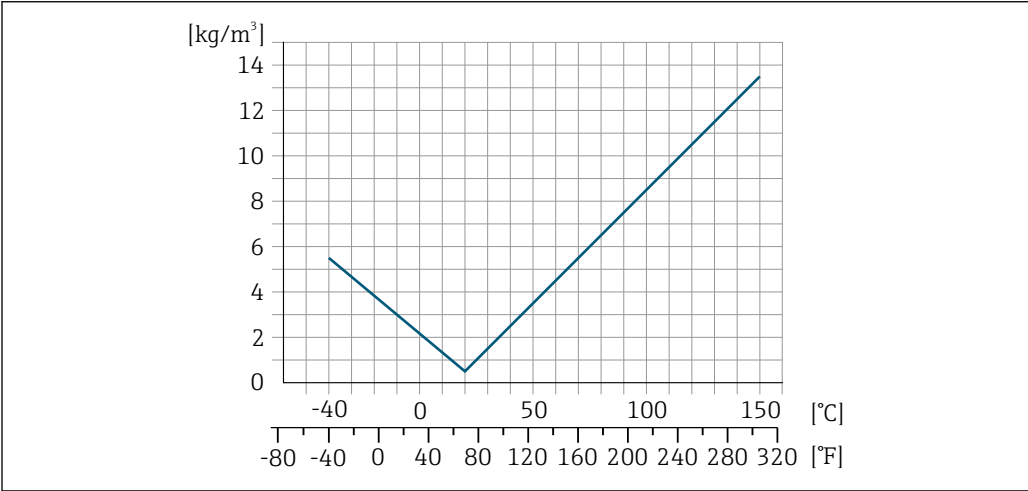
图 15 现场密度校正，例如在+20 °C (+68 °F)时
