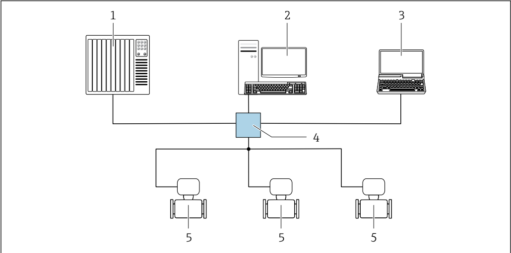
图 17 通过 EtherNet/IP 网络进行远程操作：星形拓扑结构
