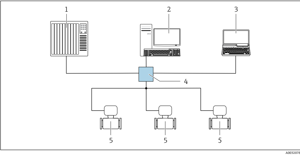
图 13 通过 EtherNet/IP 网络进行远程操作：星形拓扑结构
