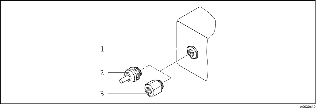
图 16 允许的电缆入口/缆塞
