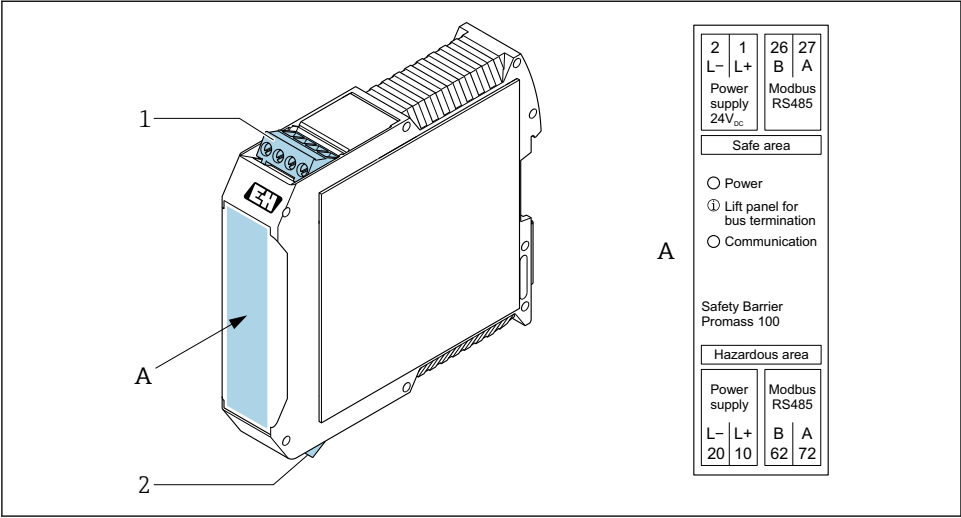
图 2 Promass 100 安全栅，带接线端子
