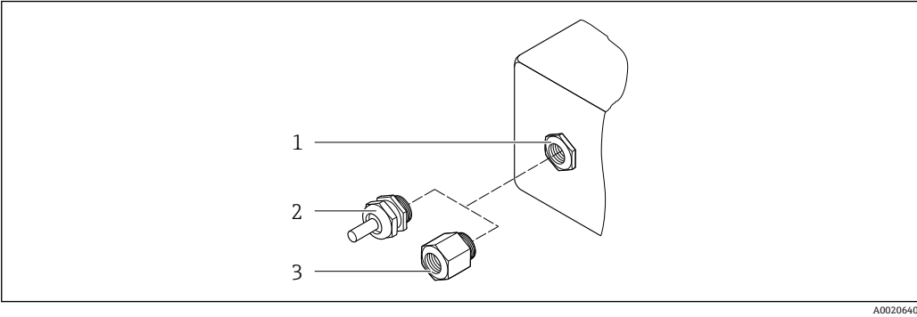
图 14 允许的电缆入口/缆塞 1 内螺纹 M20 × 1.5 2 缆塞 M20 × 1.5 3 转接头, 适用 G ½"或 NPT ½"内螺纹电缆入口
