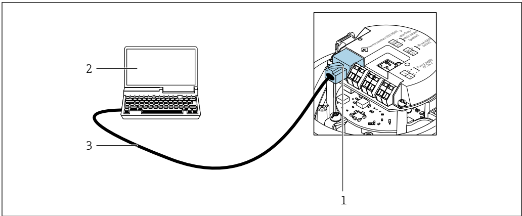
21 订购选项“输出”，选型代号 B: 4...20 mA HART，脉冲/频率/开关量输出
