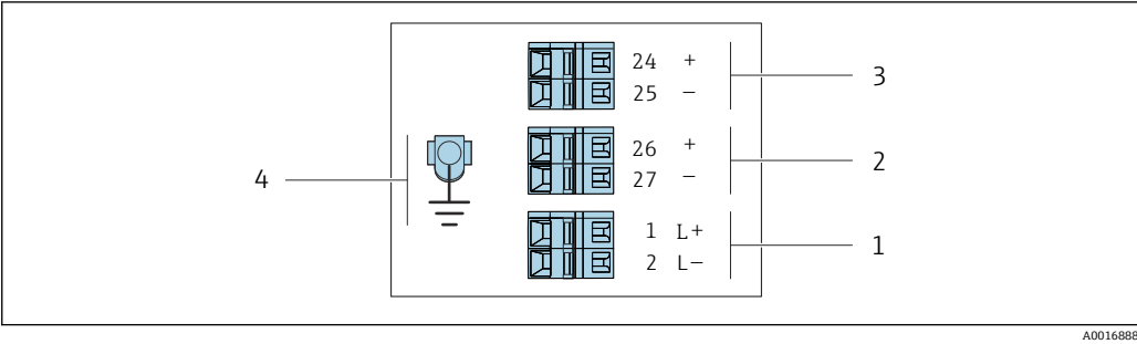
图 7 接线端子分配: 4...20 mA HART 或脉冲/频率/开关量输出
