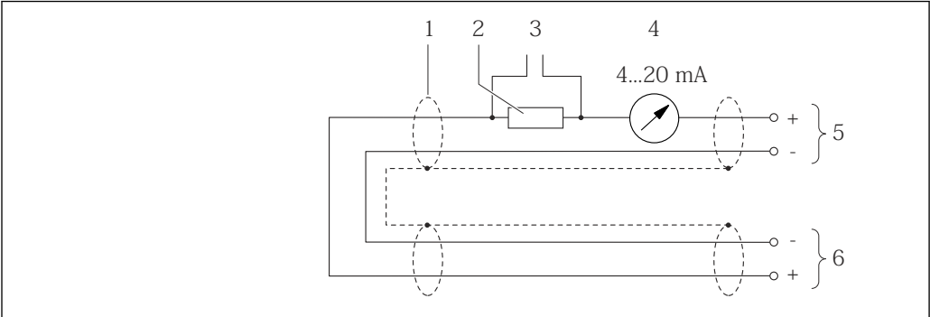
图 14 接线示例：HART 电流输入（burst 模式），HART 电流输出（有源信号）
