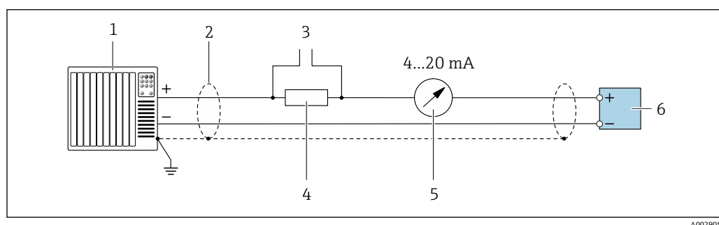
10 4...20 mA HART 电流输出 (有源) 的接线图
