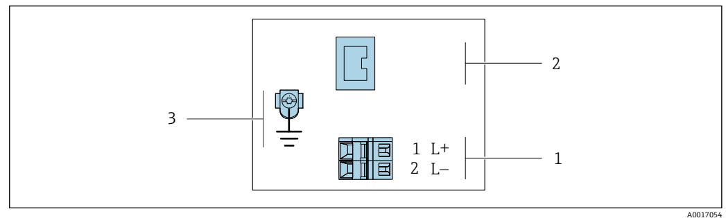
7 PROFINET 型仪表的接线端子分配
