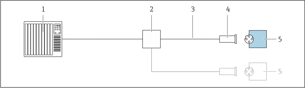
10 接线实例: PROFINET
