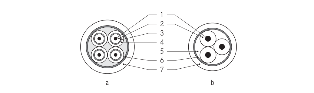
a Câble de signal b Câble de bobine
