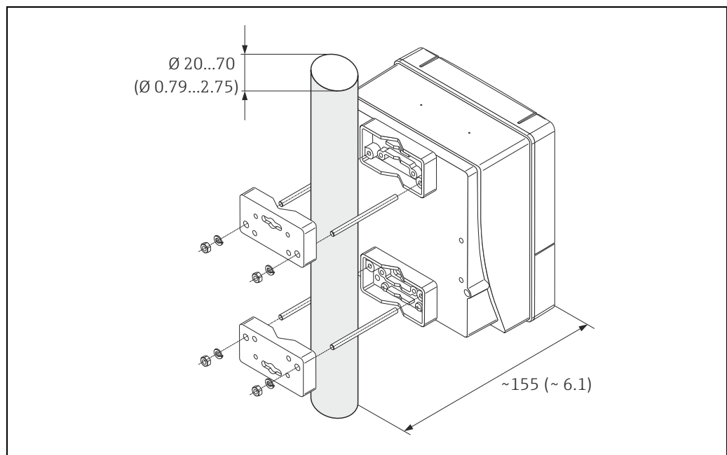
Montage sur colonne
