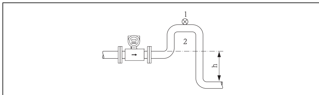
Conditions d'implantation dans le cas d'écoulements gravitaires
