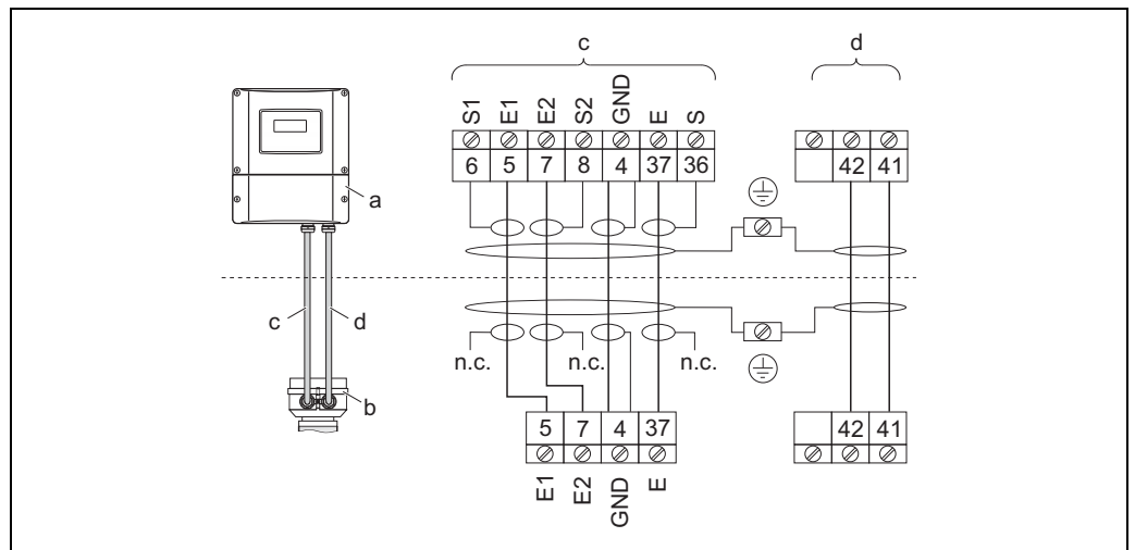
Raccordement de la version séparée
