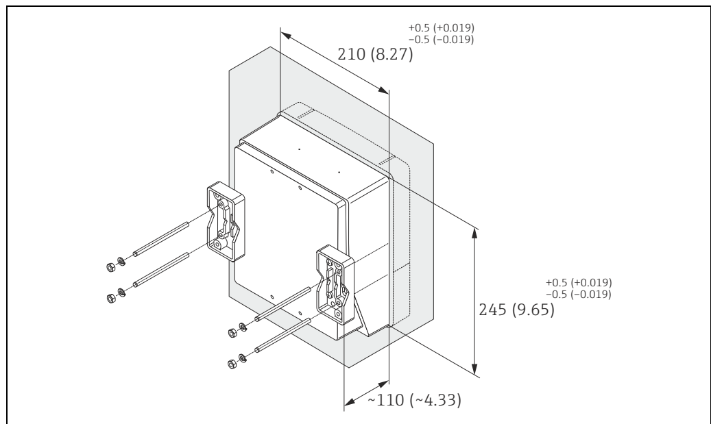
Montage en armoire électrique
