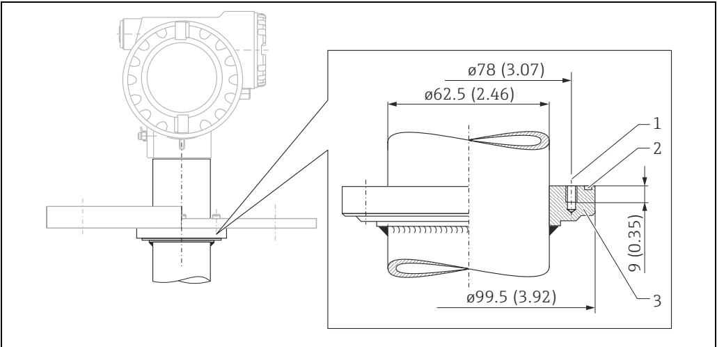
Moyeu-bride pour le montage de brides par le client. Unité de mesure mm (in)
