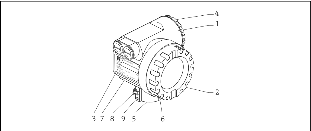
Boîtier T12 (aluminium)
