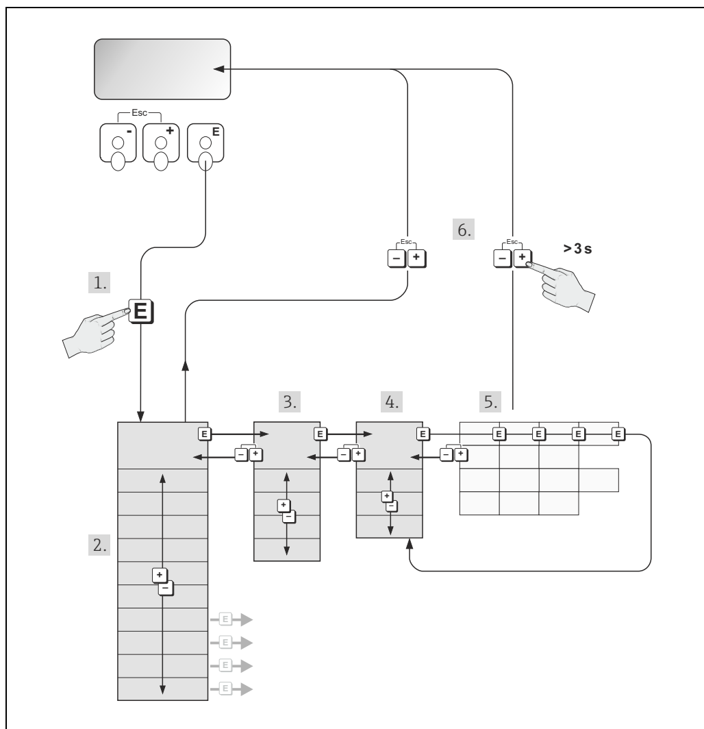
图 45: 选择功能参数和设置参数 ( 功能菜单 )
