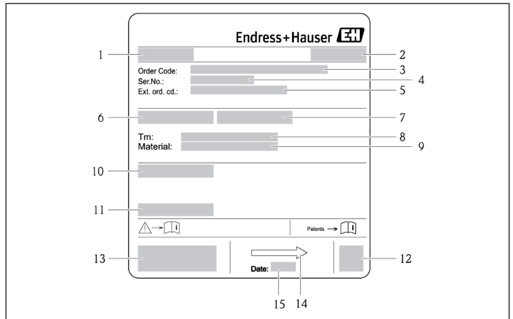
3 Образец заводской таблички сенсора
