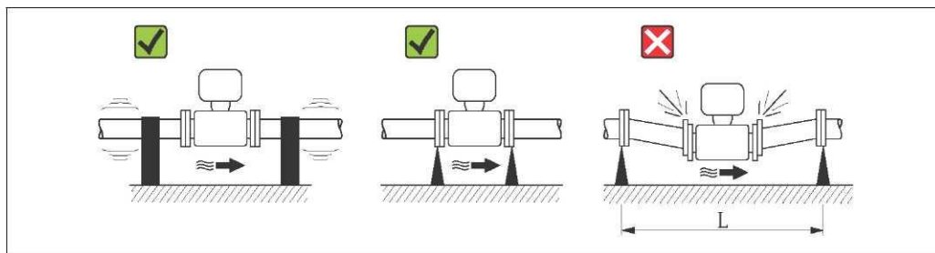
5 Меры по предотвращению вибрации прибора ( L > 10 м)
