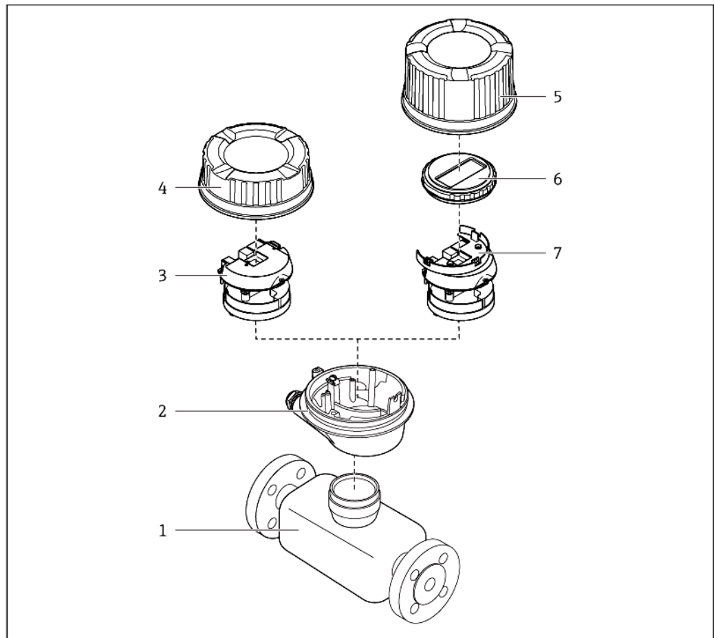
1 Важные компоненты измерительного прибора
