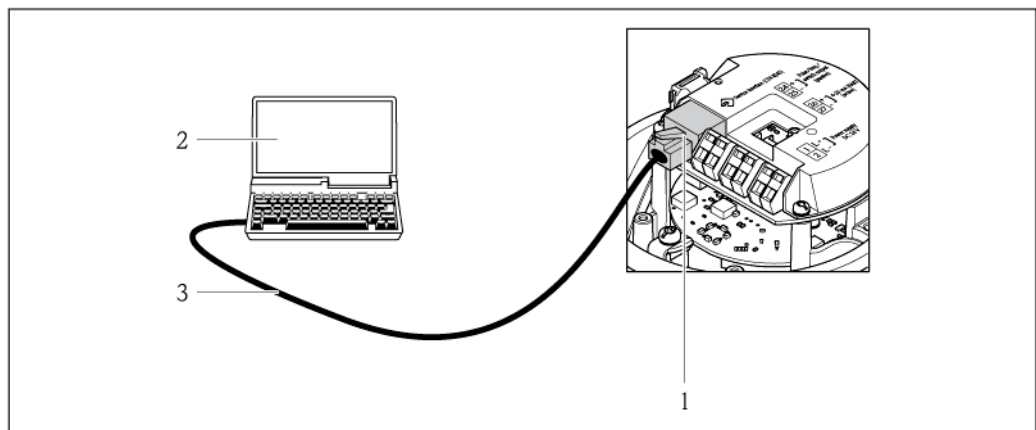
19 Подключение для кода заказа "Выход"1, опция В: 4...20 мА HART, импульсный/частотный/релейный выход
