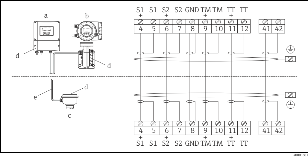
分体式仪表的电气连接示意图 a 墙装型外壳：非危险区和 ATEX II3G, 2 区防爆场合→参考防爆手册 b 墙装型外壳：ATEX II2G, 1 区 /FM/CSA 防爆场合→参考防爆手册 c 传感器接线盒 d 接线腔盖或连接外壳盖 e 连接电缆 接线端子号：4/5 = 灰；6/7 = 绿；8 = 黄；9/10 = 粉；11/12 = 白；41/42 = 棕
