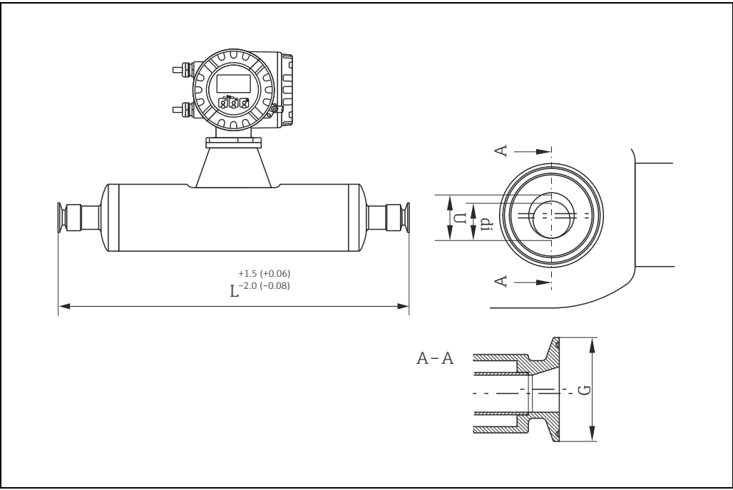
非对称 Tri-Clamp 卡箍，DIN 11866 line C
