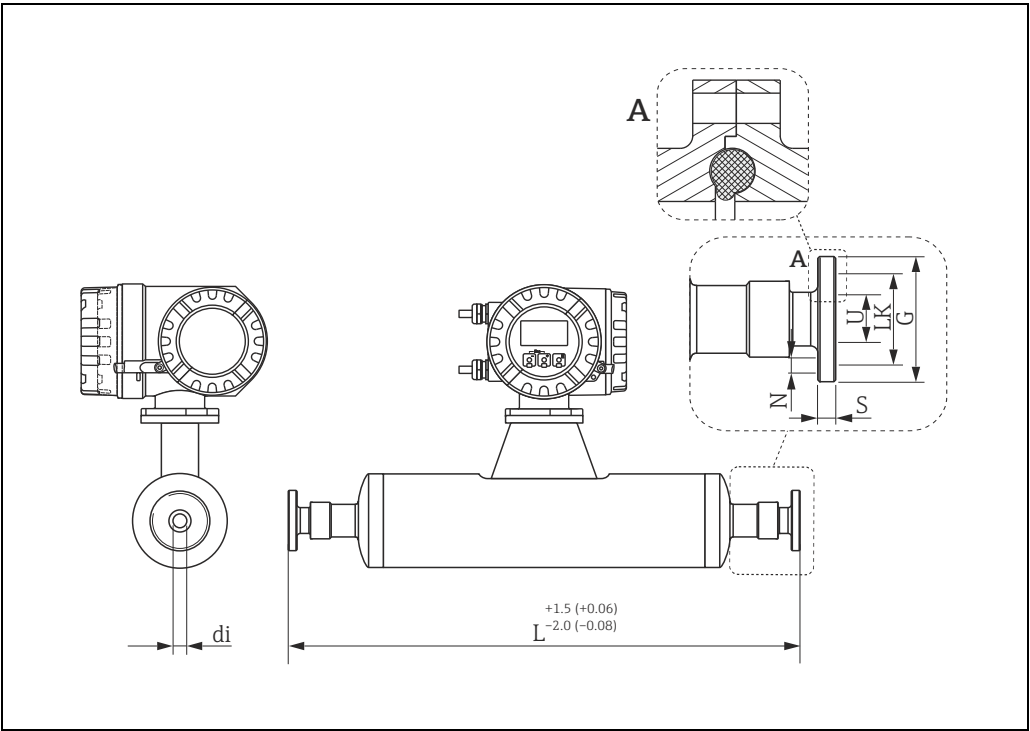
视图 A：传感器侧的槽面较小，用于在传感器侧安装 O 型圈。安装传感器时，配套法兰应具有较大的槽面。单位：mm (in)
