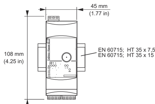
Abb. 4-1: Maße des Fieldgates FXA320
