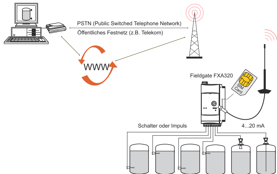
Abb. 3-5: Fieldgate mit einem Mobilfunknetz verbinden
