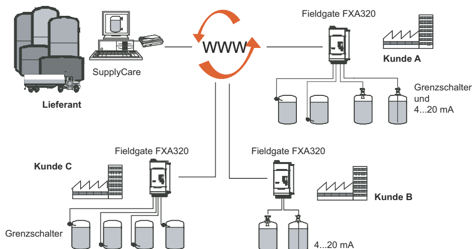
Abb. 3-1: Bestandsüberwachung mit Fieldgate FXA320
