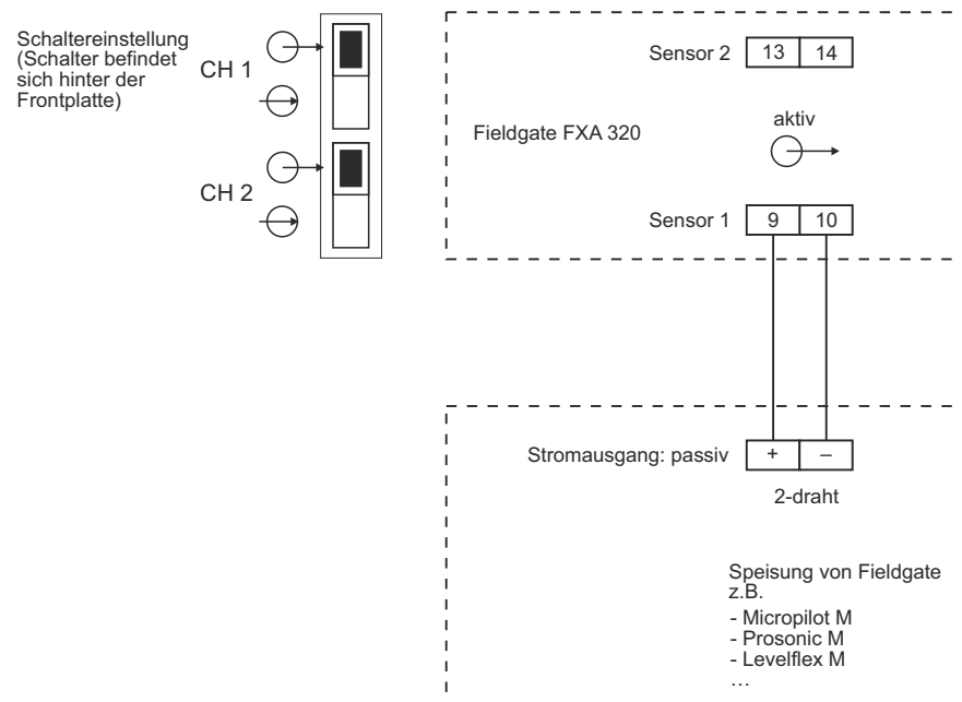
Abb. 4-7: Verdrahtung für passive 4...20 mA-Geräte
