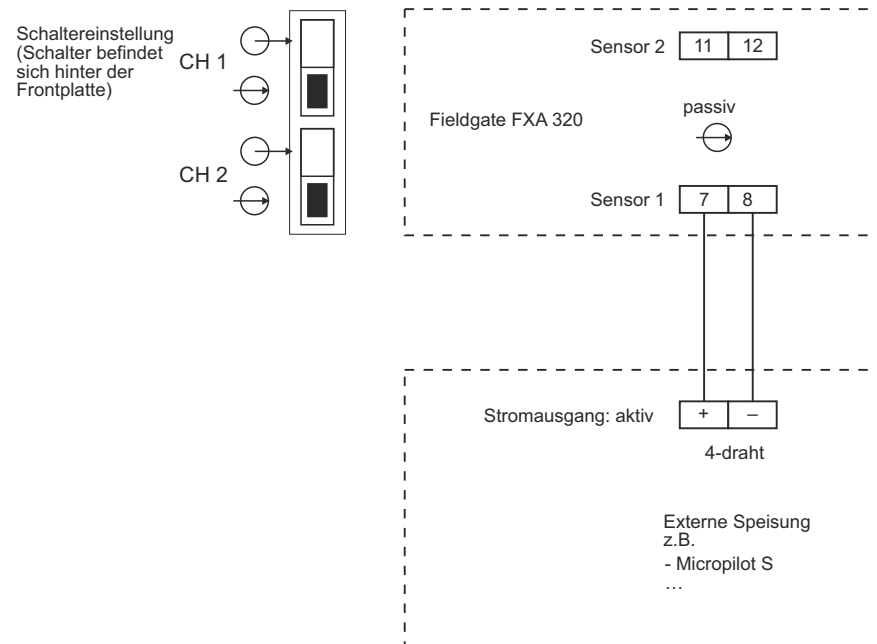
Abb. 4-6: Verdrahtung für aktive 4...20 mA-Geräte
