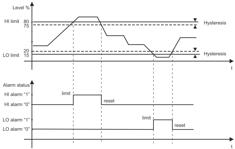
Abb. 6-2: Beispiel für Füllstand-Grenzwerte und Hysteresis
