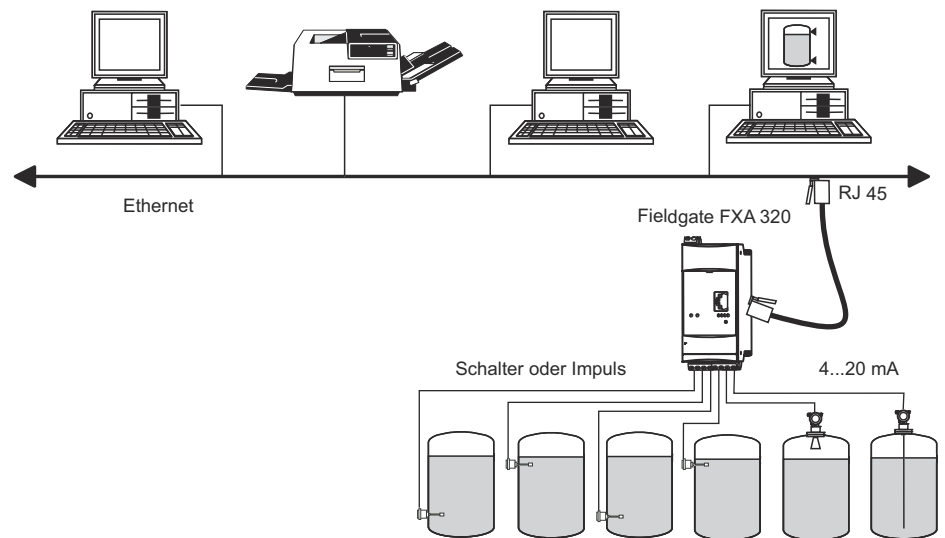
Abb. 3-3: Fieldgate mit Ethernet verbinden
