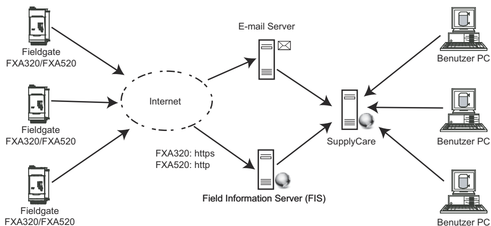
Abb. 3-2: Bestandsüberwachung mittels E-mail-Server bzw. FIS
