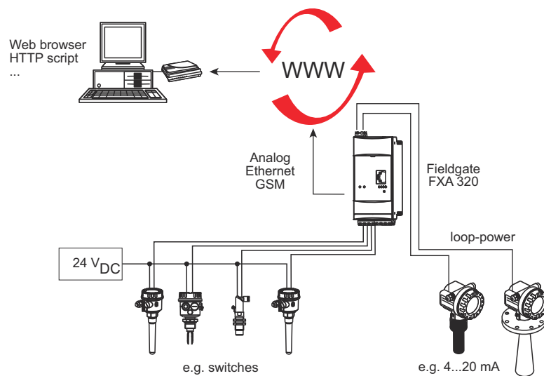
Abb. 3-8: Systemaufbau für 4...20 mA- und Digitalanschlüsse
