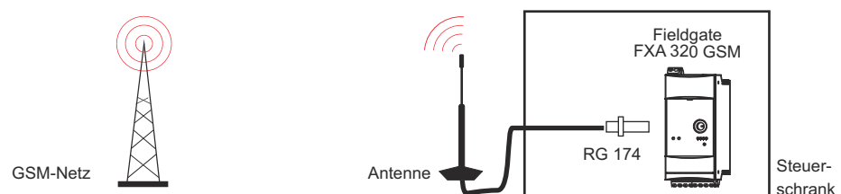
Abb. 4-11: Anschluss des Fieldgates an ein GSM-Netz
