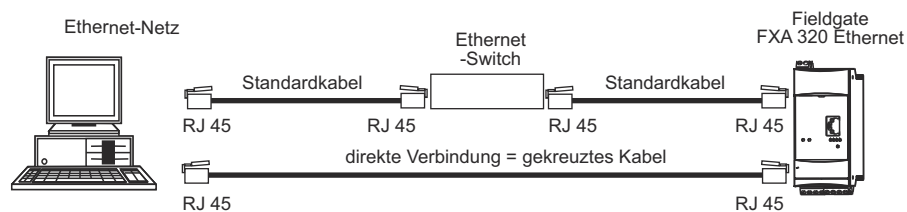
Abb. 4-10: Anschluss des Fieldgates an ein Ethernet-Netz
