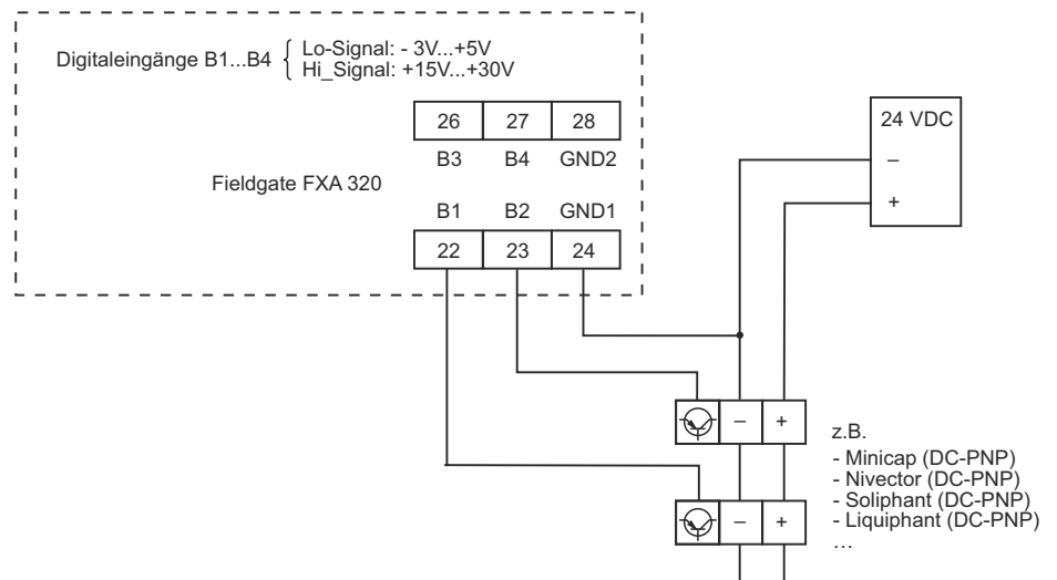
Abb. 4-8: Verdrahtung der optionalen Digitaleingängen
