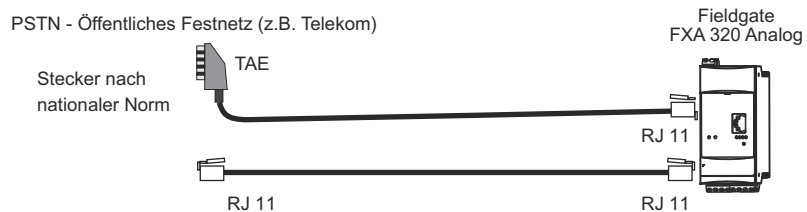
Abb. 4-9: Anschluss von Fieldgate ans leitungsvermittelte Telefonnetz
