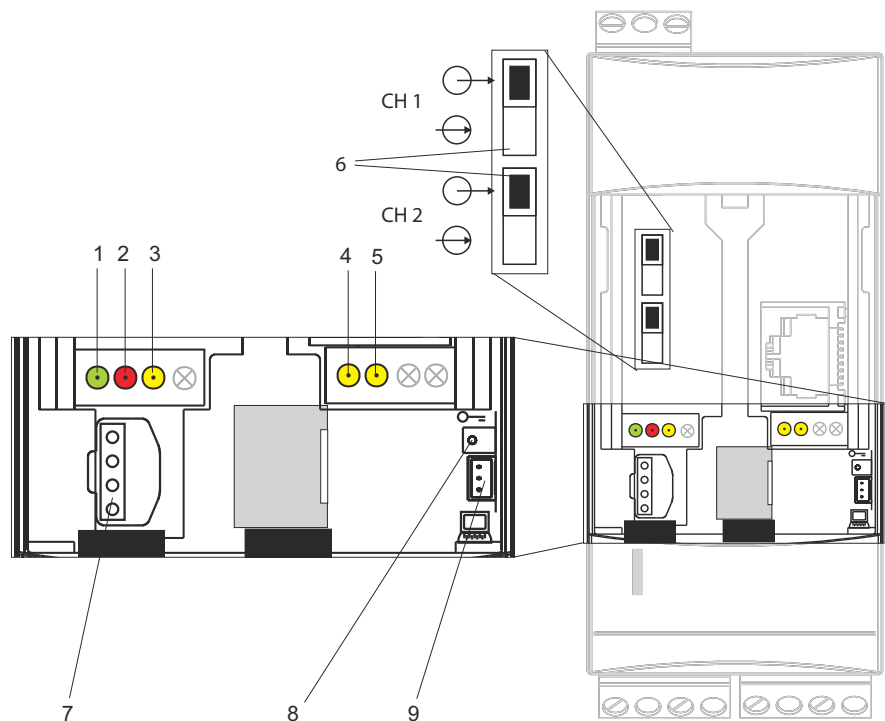
Abb. 3-6: Frontplatte des Fieldgates FXA320
