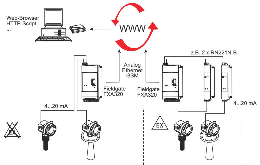
Abb. 3-7: Systemaufbau für 4...20 mA-Anschlüsse
