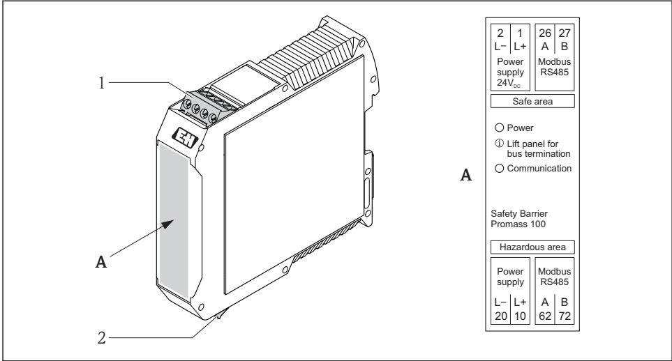
10 Barrera de seguridad Promass 100 con terminales
