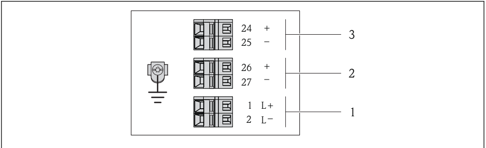
5 Asignación de terminales 4-20 mA HART, salida de impulsos/frecuencia/conmutación
