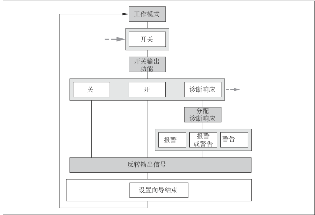
图 22 “脉冲/频率/开关 输出” 向导，在“设置” 菜单“工作模式” 参数“开关” 选项 1 中(第一部分)
