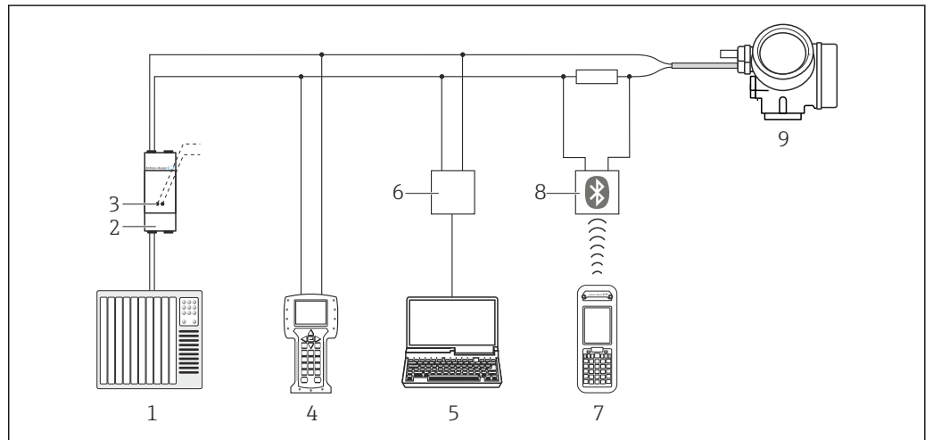
图 37 通过 HART 通信进行远程操作
