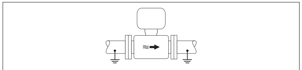
6 通过测量管实现电势平衡
