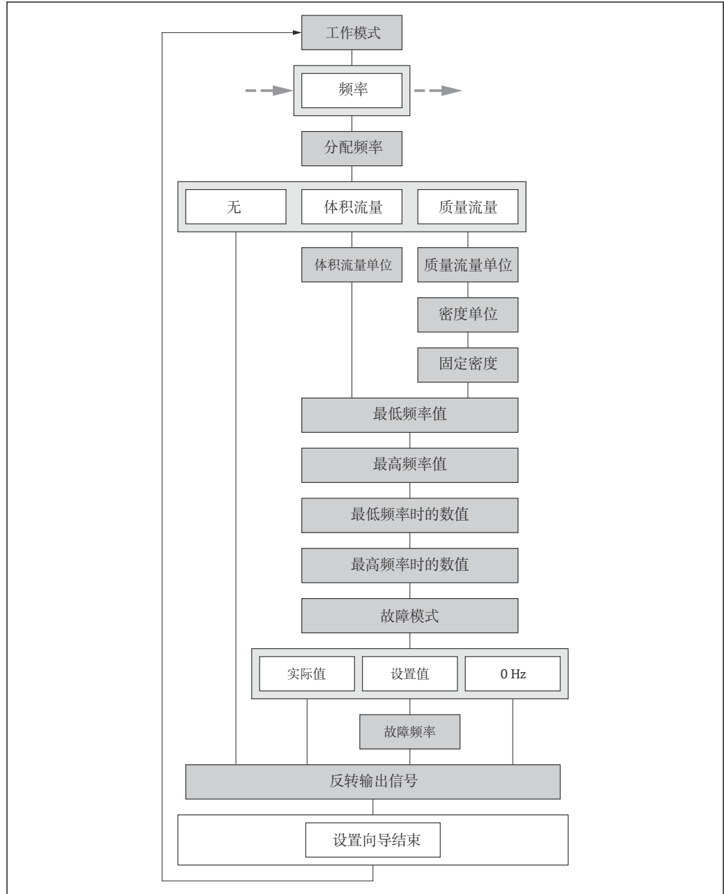
图 21 “脉冲/频率/开关 输出” 向导，在“设置” 菜单：“工作模式” 参数“频率” 选项中
