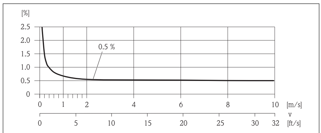
图 34 最大测量误差(% o.r.)示意图
