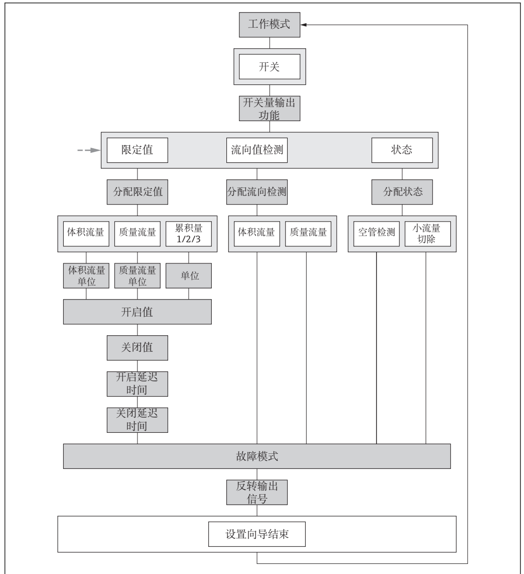
图 23 “脉冲/频率/开关 输出”向导，在“设置”菜单“工作模式”参数“开关”选项 2 中(第二部分)
