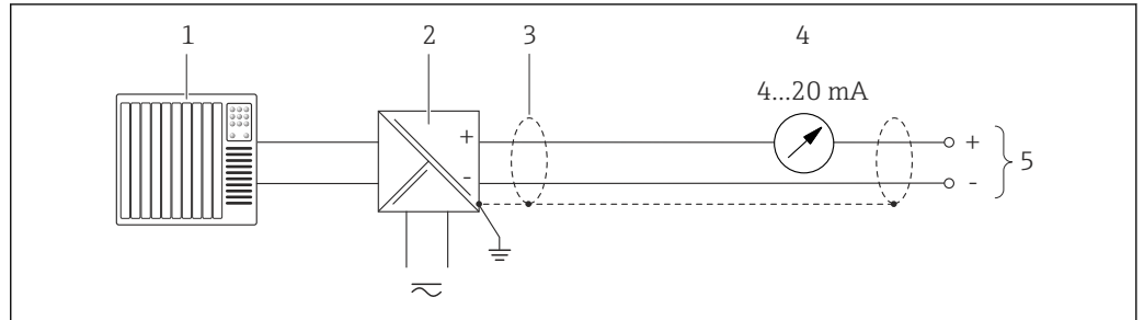
图 9 4...20 mA HART 无源电流输出的连接示例
