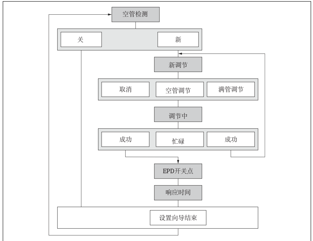
图 27 “空管检测” 向导，在“设置” 菜单中
