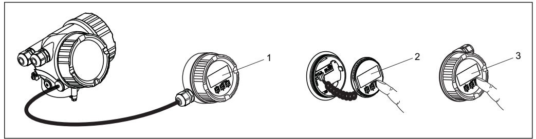
图 36 通过 FHX50 操作的操作选项
