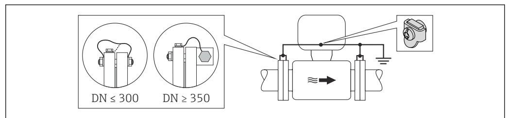
7 通过接地端子和管道法兰实现系统电势平衡
