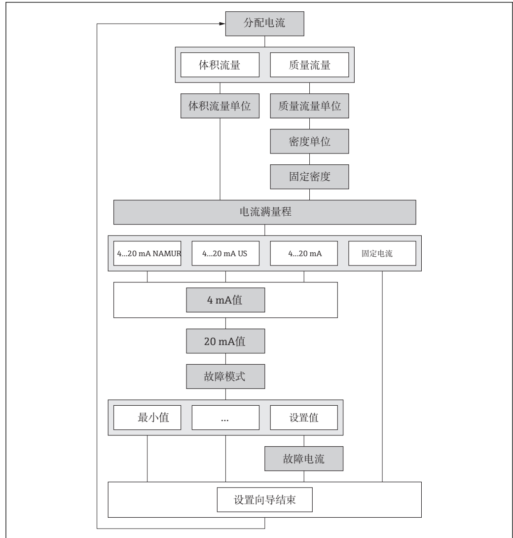
图 19 “电流输出 1” 向导，在“设置”菜单中
