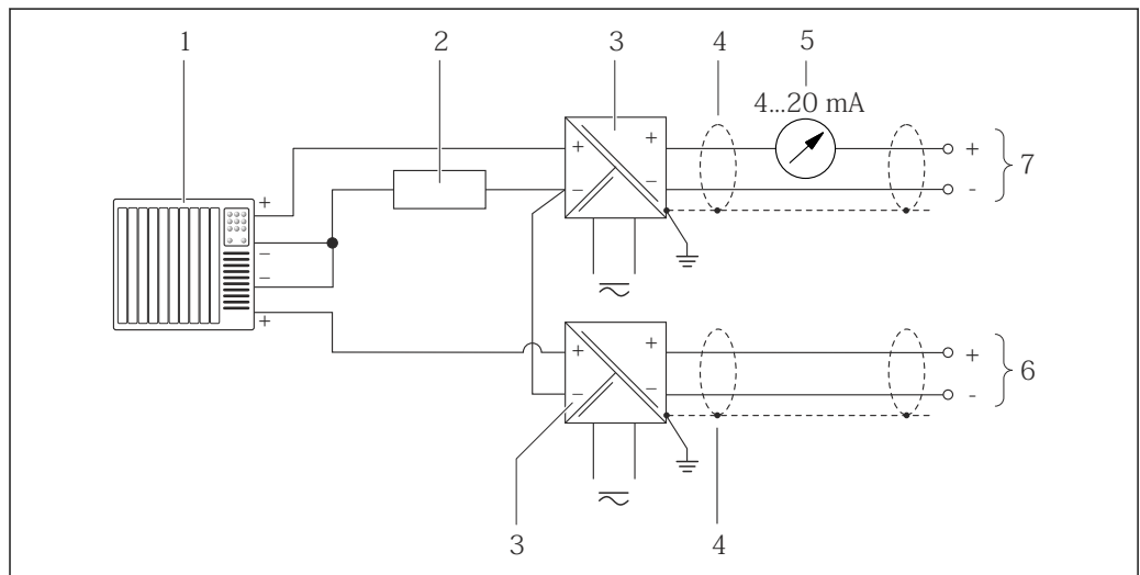
图 12 HART 输入(共用负信号端)的连接示意图
