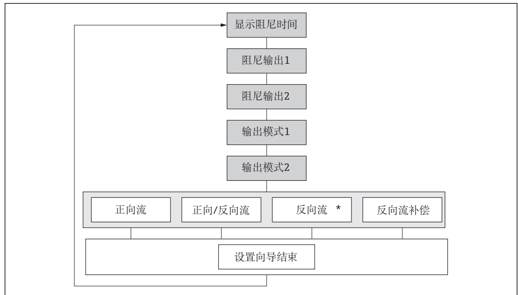
图 25 “输出设置” 向导，在“设置” 菜单中
