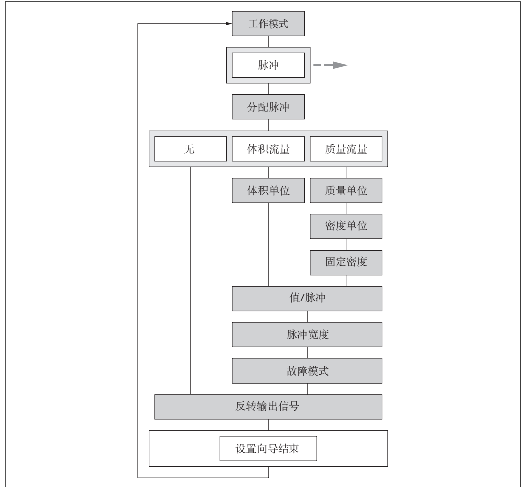
图 20 “脉冲/频率/开关 输出” 向导，在“设置” 菜单中：“工作模式” 参数“脉冲” 选项
