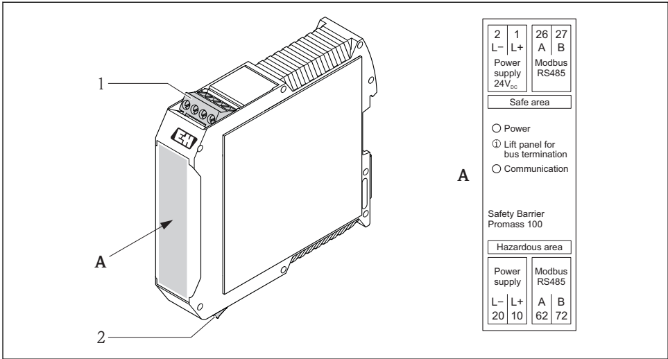
图 10 Promass 100 安全栅和接线端子示意图
