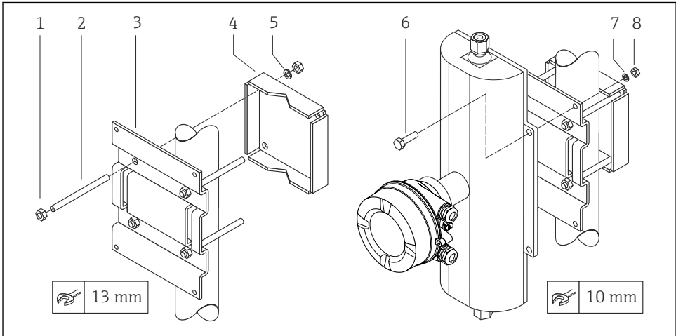
图 4 柱式安装套件示意图
