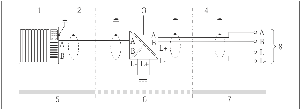
图 13 变压器和 Promass 100 安全栅间的电气连接
