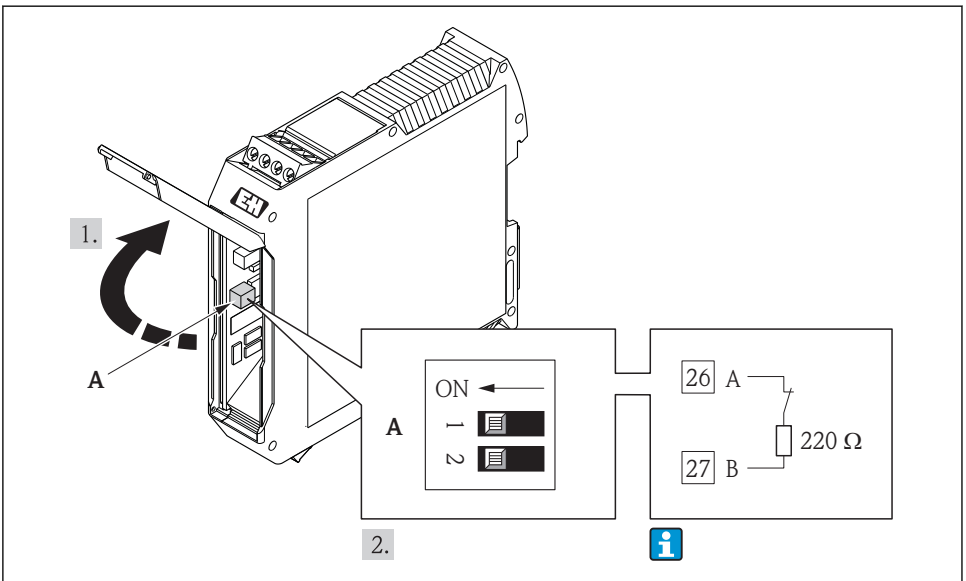
☑ 17 通过 Promass 100 安全栅上的 DIP 开关开启终端电阻
