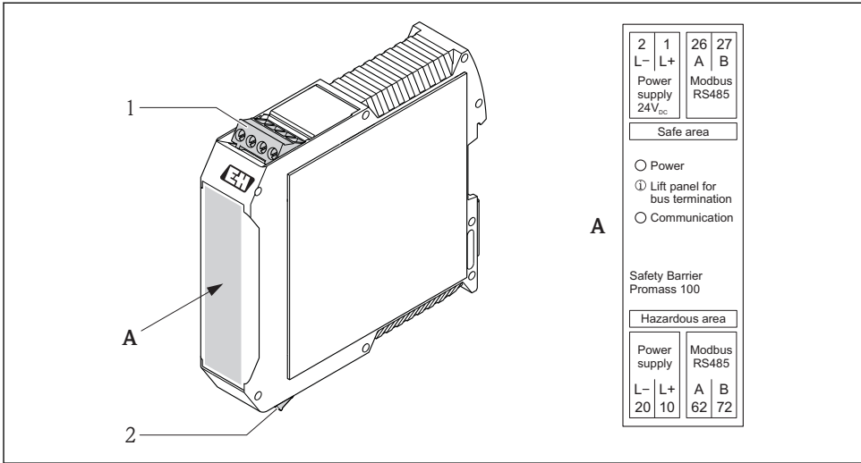
图 10 Promass 100 安全栅和接线端子示意图
