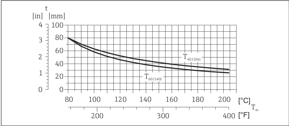
图 4 最大推荐保温层厚度取决于介质温度和环境温度
