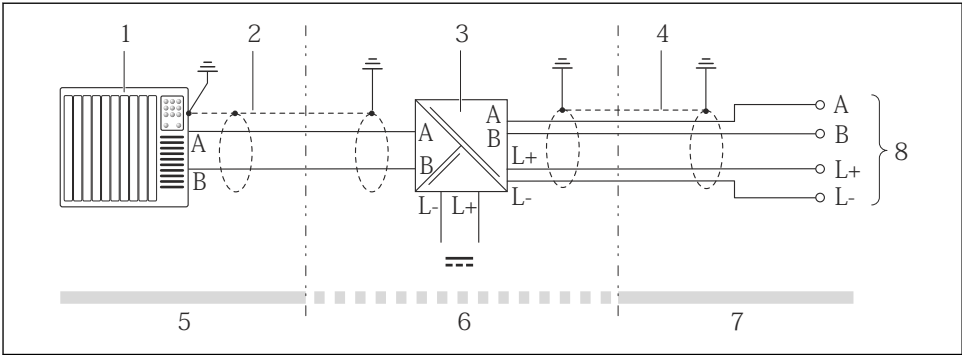
14 Raccordement électrique entre le transmetteur et la barrière de sécurité Promass 100
