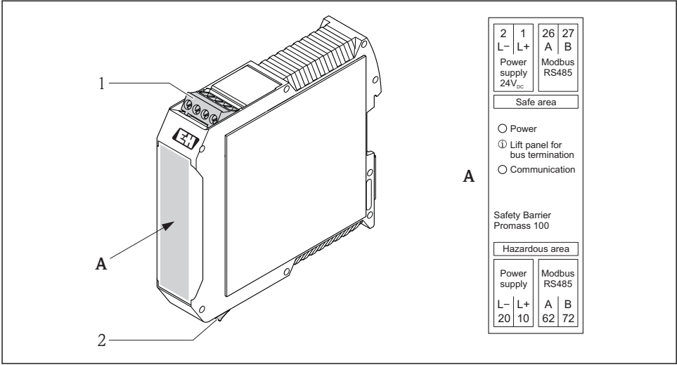
11 Barrière de sécurité Promass 100 avec raccords
