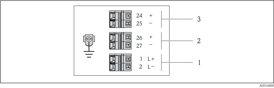
6 Occupation des bornes 4-20 mA HART avec sortie impulsion/fréquence/tor
