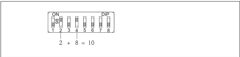
图 5 硬件地址设定实例。开关 8 放置在“OFF (关)”位置上，开关 1...7 确定设备地址。
