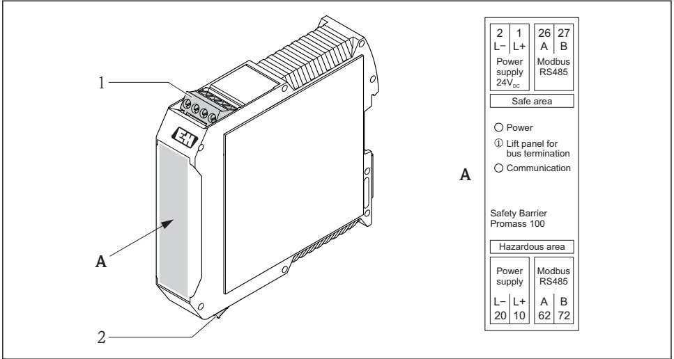
图 5 Promass 100 安全栅和接线端子示意图
