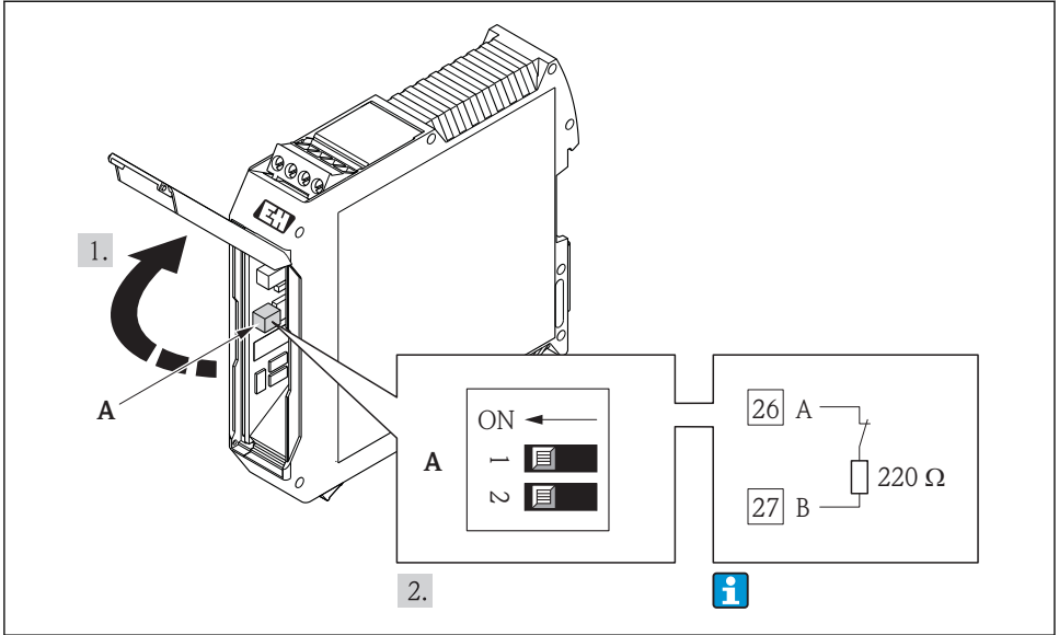
图 9 通过 Promass 100 安全栅上的 DIP 开关开启终端电阻
