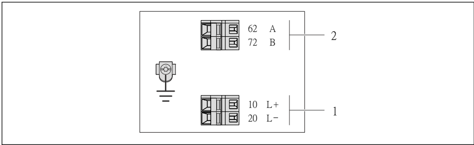
图 4 Modbus RS485 型仪表的接线端子分配示意图, 连接类型适用于在本安防爆场合中使用(通过 Promass 100 安全栅连接)
