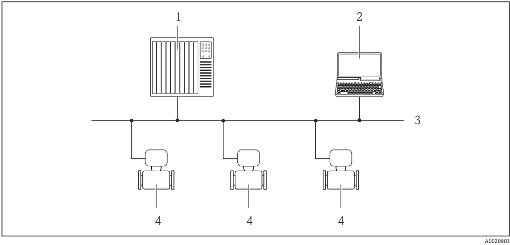
图 15 通过 PROFIBUS DP 网络进行远程操作
