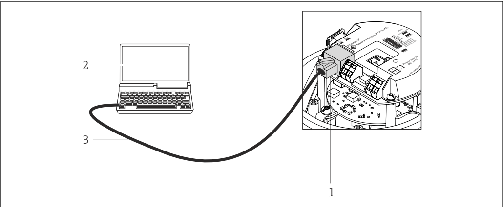
20 订购选项“输出”，选型代号 L: PROFIBUS DP 1 测量设备的服务接口 (CDI-RJ45)，内置 Web 服务器访问接口 2 计算机，带 Web 浏览器 (例如：互联网浏览器)，用于访问内置设备 Web 服务器；或安装有“FieldCare”调试工具，带 COM DTM “CDI 通信 TCP/IP” 互联网浏览器)，用于访问内置设备 Web 服务器；或安装有“FieldCare”调试工具，带 COM DTM “CDI 通信 TCP/IP” 3 标准以太网连接电缆，带 RJ45 插头
