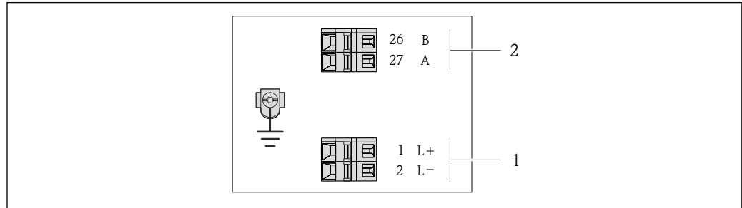
图 8 PROFIBUS DP 型仪表的接线端子分配示意图
