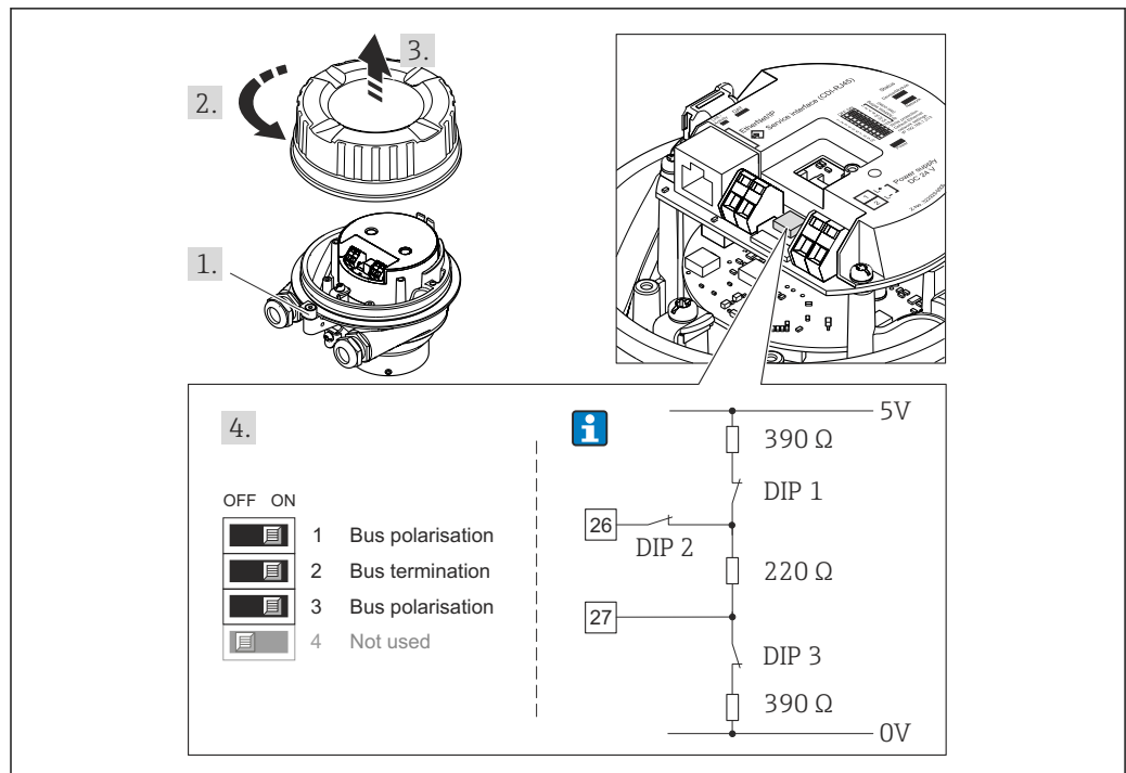
图 13 使用 I/O 电子模块上的 DIP 开关端接(波特率小于 1.5 MBaud)
