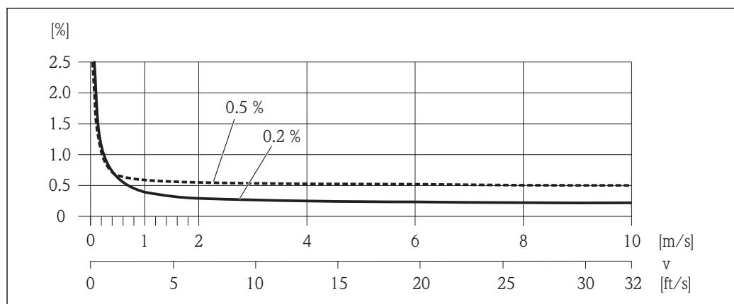
图 18 最大测量误差(% o.r.)示意图
