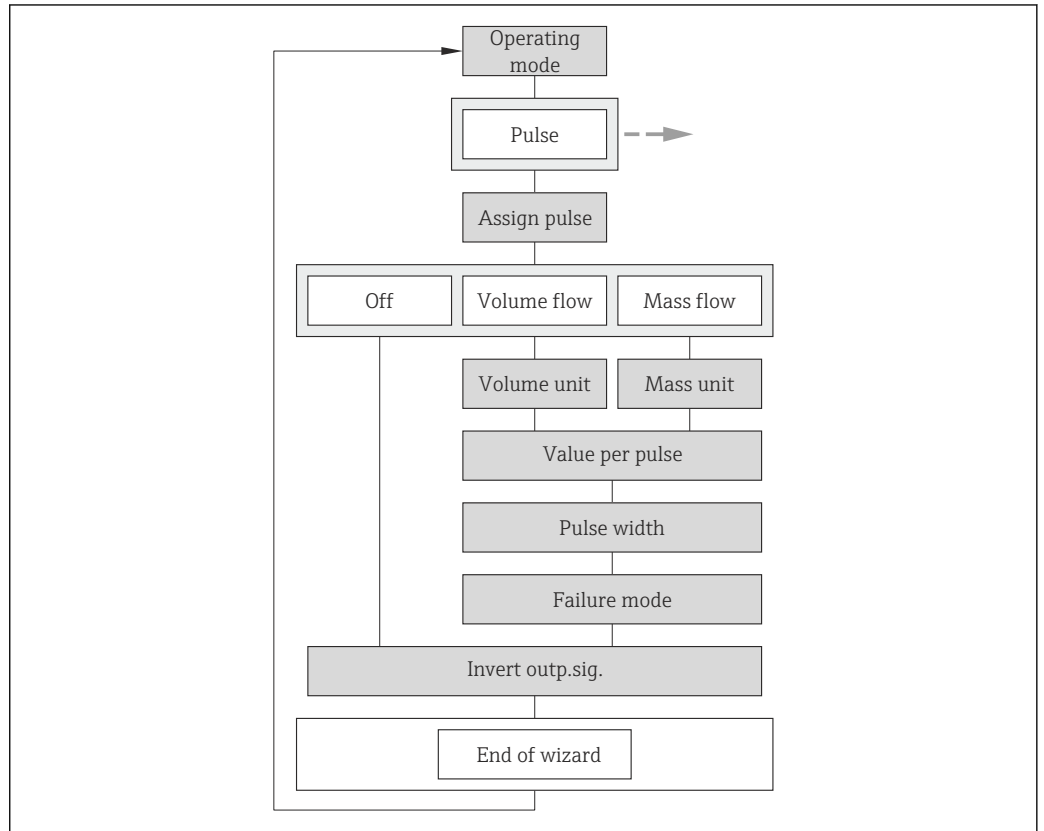
图 13 “脉冲/频率/开关 输出” 向导，在“高级设置”子菜单中：“工作模式”参数“脉冲”选项
