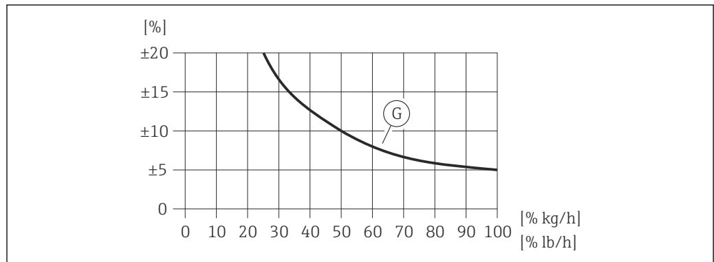
图 23 最大测量误差(%质量流量), 参考下表订购选项“标定流量”, 选型代号 G (未验证); 请参考下表
