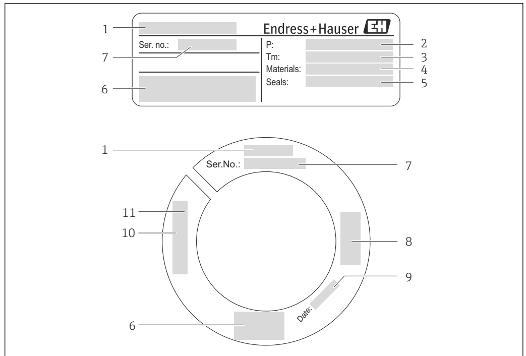
图 2 传感器的铭牌示意图
