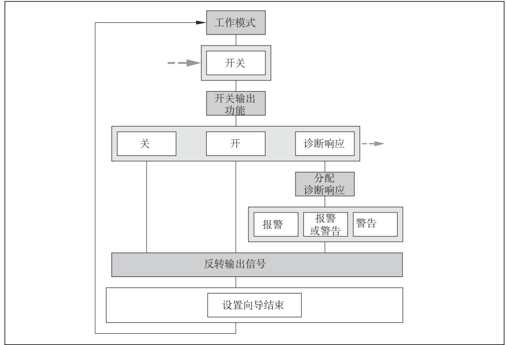
图 15 “脉冲/频率/开关 输出” 向导，在“高级设置”子菜单中：“工作模式”参数“开关”选项中(第一部分)
