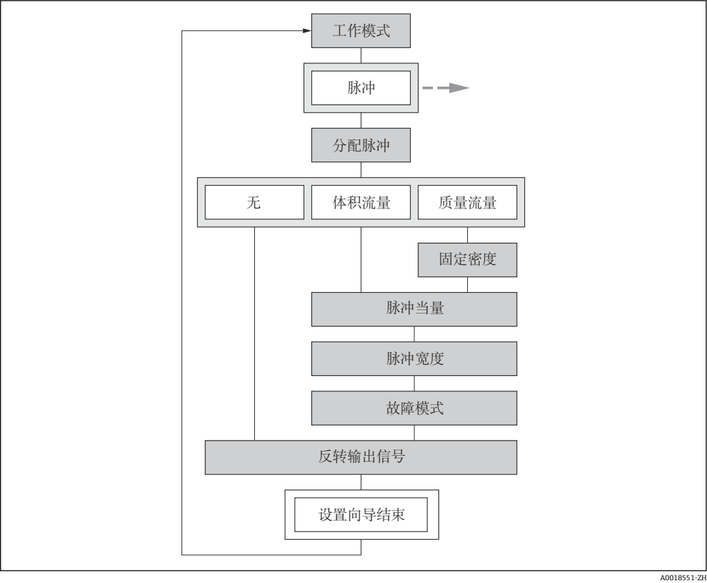
图 22 “脉冲/频率/开关 输出” 向导，在“设置” 菜单中：“工作模式” 参数“脉冲” 选项
