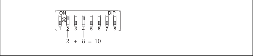
图 11 硬件地址设定实例。开关 8 放置在“OFF (关)”位置上，开关 1...7 确定设备地址。
