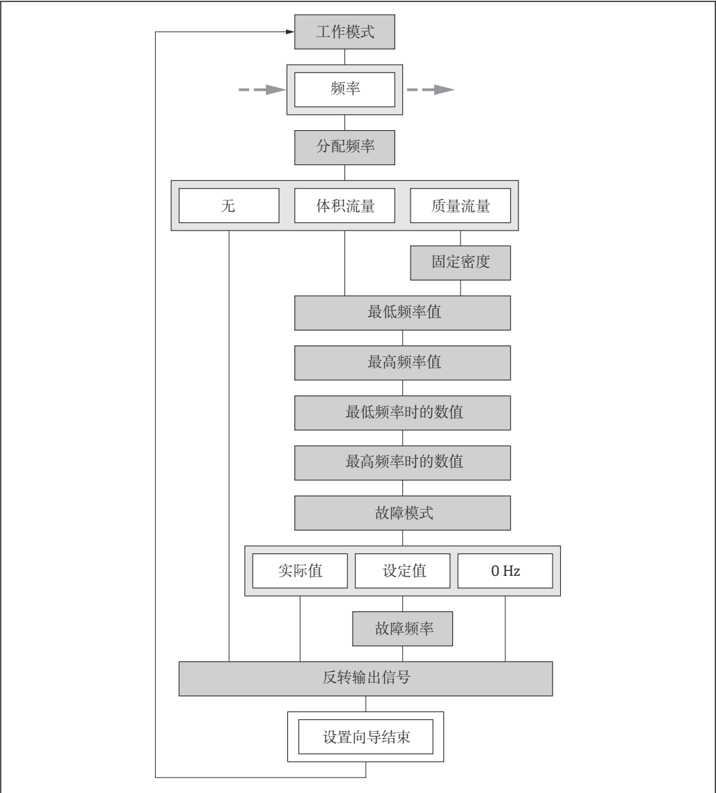
图 23 “脉冲/频率/开关 输出” 向导，在“高级设置” 子菜单中：“工作模式” 参数“频率” 选项
