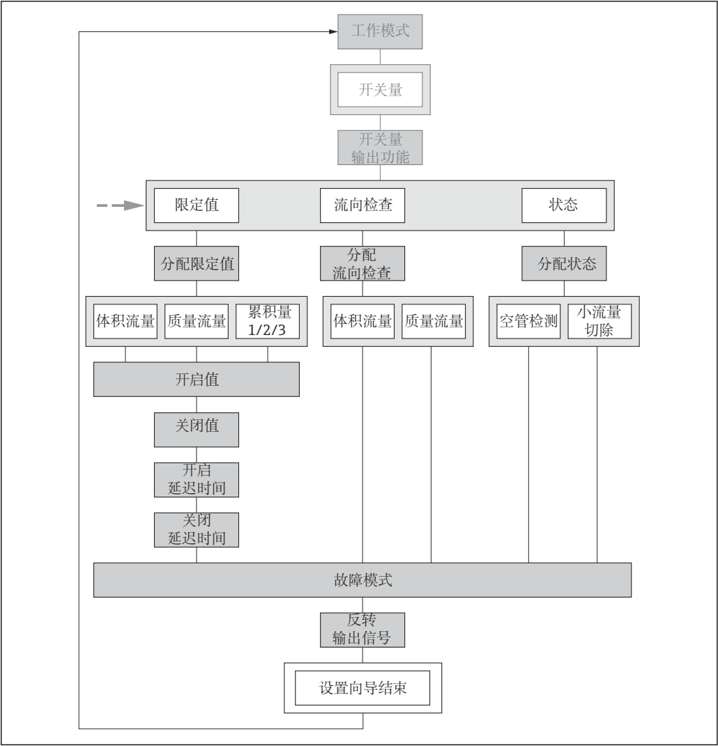
图 25 “脉冲/频率/开关 输出”向导，在“高级设置”子菜单中：“工作模式”参数“开关”选项(第二部分)
