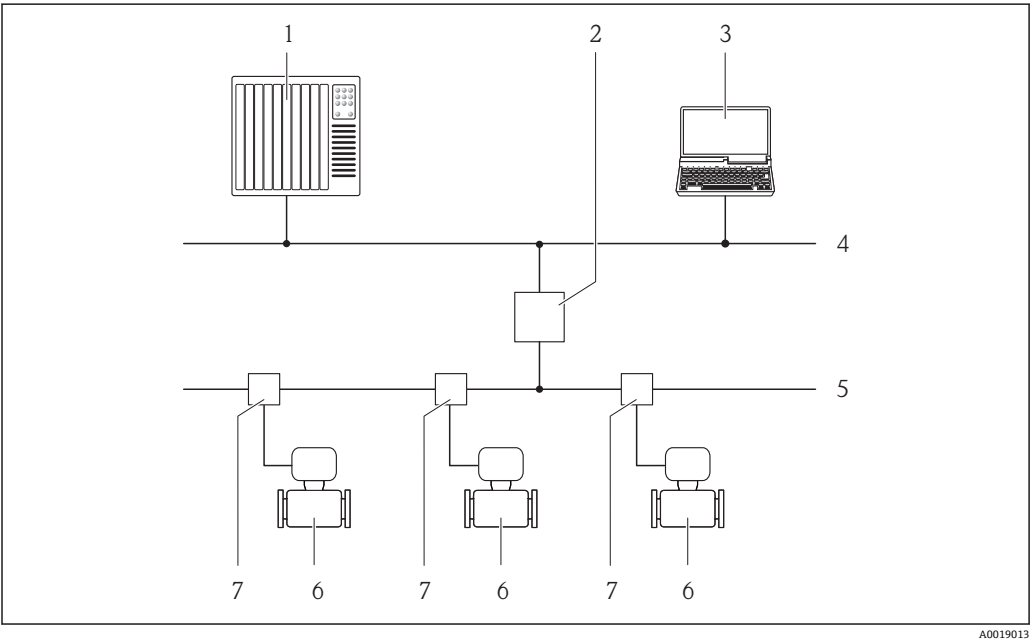
35 通过 PROFIBUS PA 网络进行远程操作 1 自动化系统 2 PROFIBUS DP/PA 段耦合器 3 带 PROFIBUS 网络卡的计算机 4 PROFIBUS DP 网络 5 PROFIBUS PA 网络 6 测量设备 7 T 型盒
