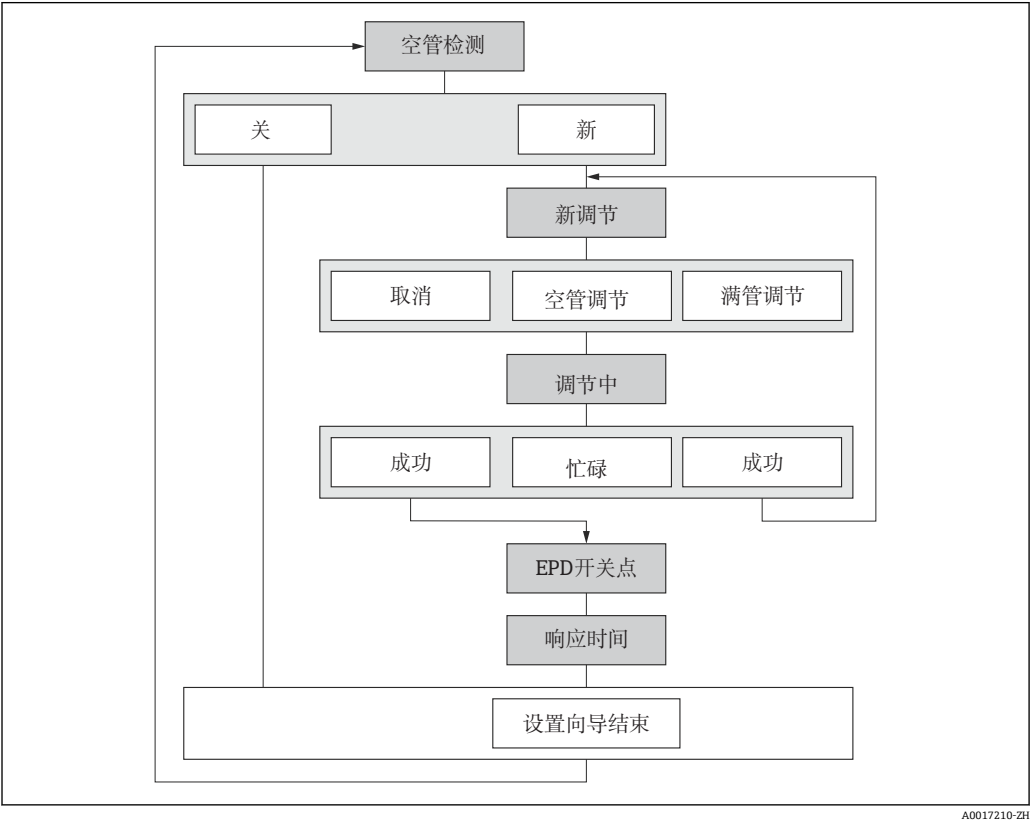
图 21 “空管检测” 向导，在“设置” 菜单中
