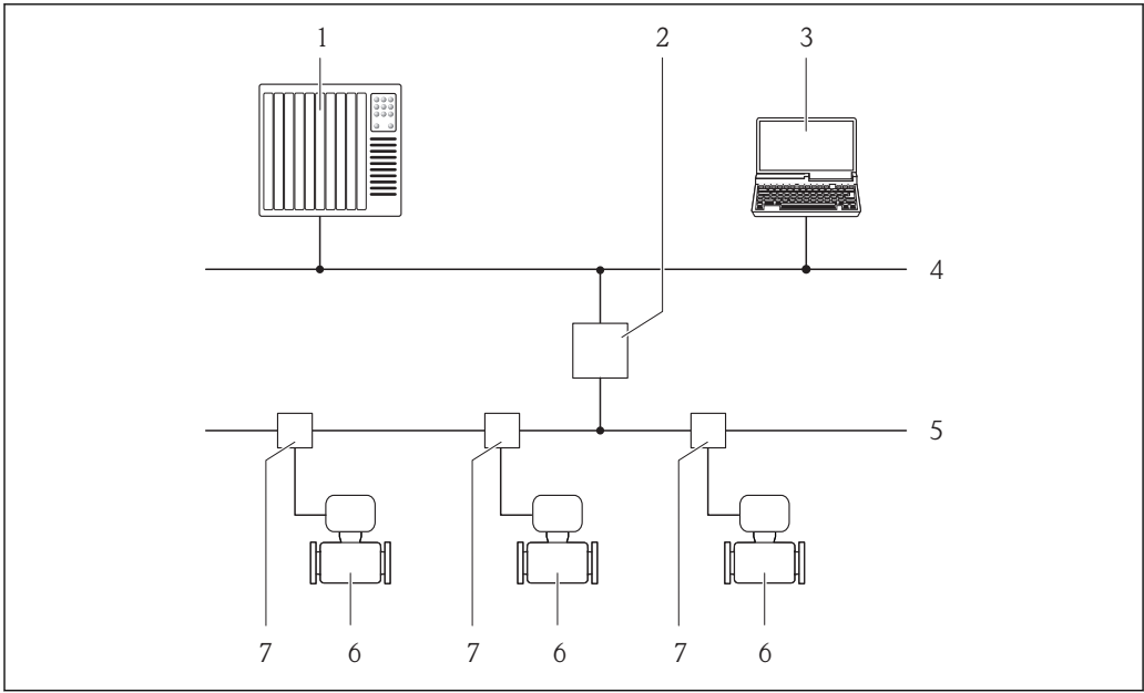
15 通过 PROFIBUS PA 网络进行远程操作
