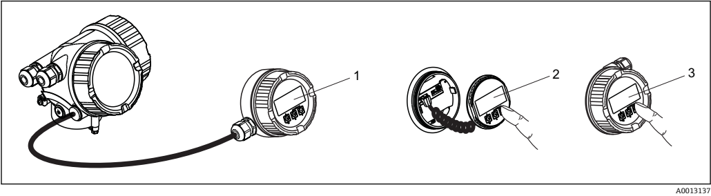
34 通过 FHX50 操作的操作选项 1 分离型显示与操作单元 FHX50 的外壳 2 SD02 显示与操作单元，按键操作；操作时必须打开盖板 3 SD03 显示与操作模块，光敏键：可以通过盖板玻璃操作
