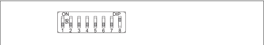
图 12 软件地址设定实例。开关 8 放置在“ON (开)”位置上；在操作菜单中设置地址(“设置” 菜单→“通信” 子菜单→“设备地址” 参数)。
