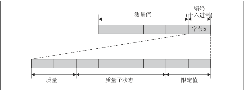
图 28 编码字节的结构
