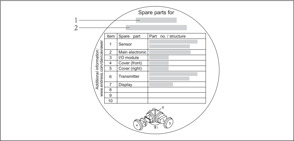
31 接线腔盖中的“备件概述图标”示例
