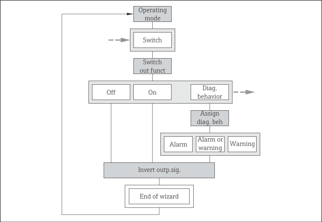
图 24 “脉冲/频率/开关 输出” 向导，在“高级设置” 子菜单中：“工作模式” 参数“开关” 选项(第一部分)
