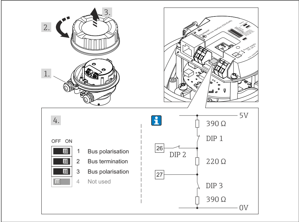
15 Terminações usando minisseletores com módulos de componentes eletrônicos E/S (para taxas de transmissão < 1.5 MBaud)
