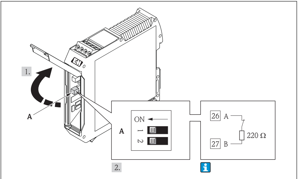
16 通过 Promass 100 安全栅上的 DIP 开关开启终端电阻
