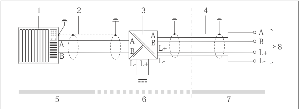
图 12 变压器和 Promass 100 安全栅间的电气连接
