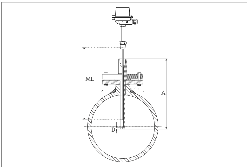
图 4 温度计的安装示意图
