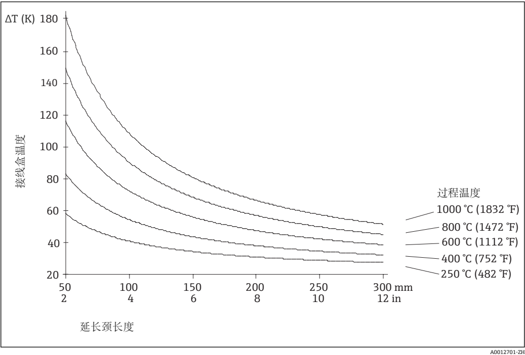
图 5 接线盒受热与延长颈长度的关系曲线。接线盒温度=环境温度 20 °C (68 °F) + ΔT
