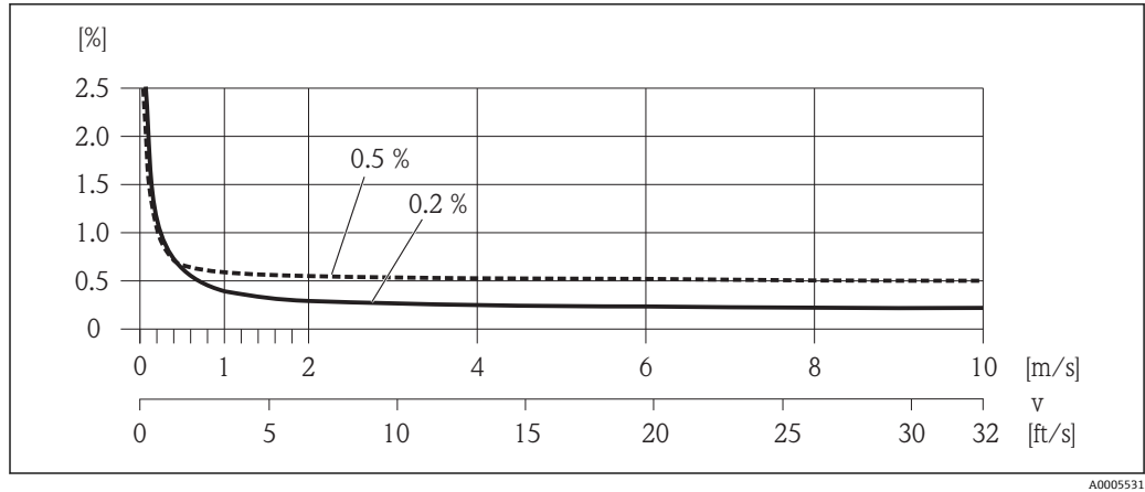
图 15 最大测量误差(% o.r.)示意图
