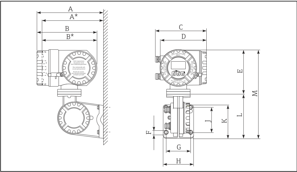
分体式仪表的变送器接线盒 (II2G/1 区防爆场合 )
