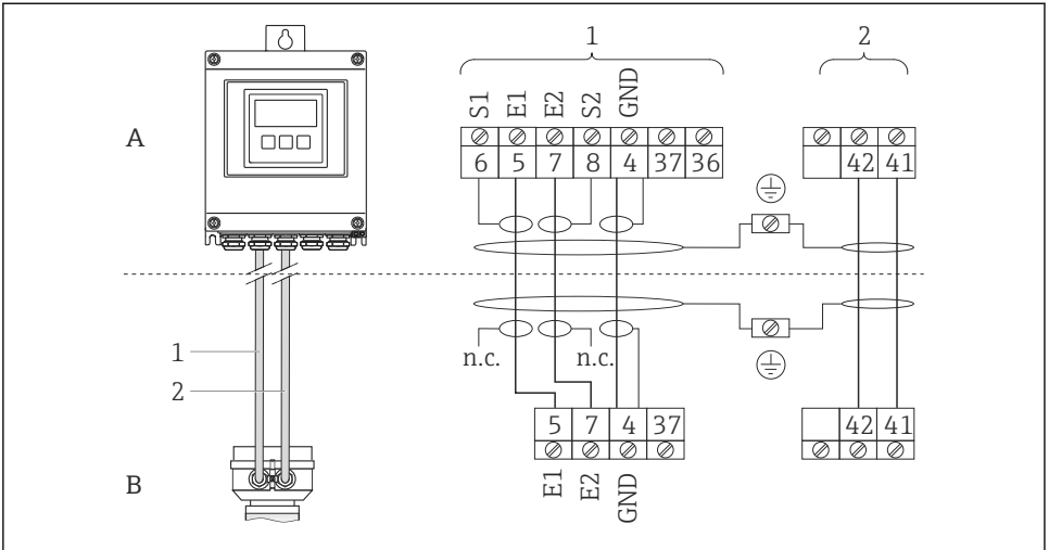
7 Esquema de ligação elétrica da versão remota
