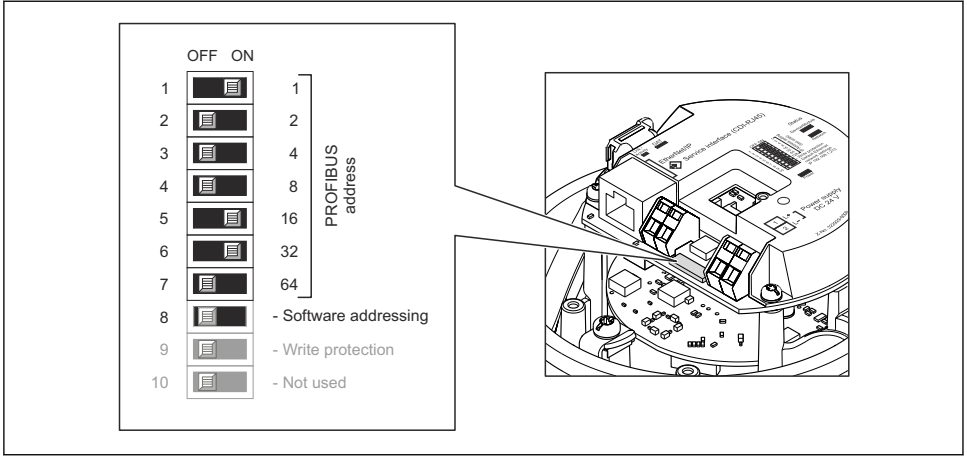
☑ 15 通过 I/O 电子模块上的 DIP 开关设定地址
