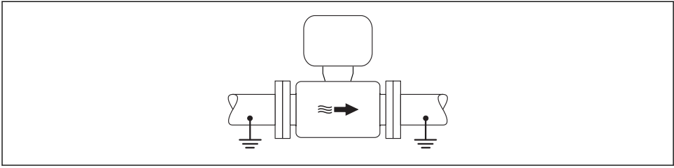
图 12 通过测量管实现电势平衡
