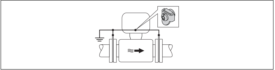
图 14 通过接地端子和接地环实现系统电势平衡
