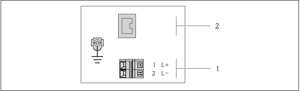
图 9 工业以太网(EtherNet/IP)的接线端子分配示意图
