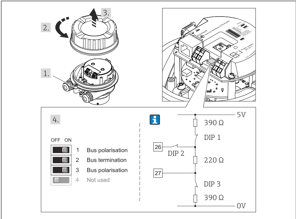
图 16 使用 I/O 电子模块上的 DIP 开关端接(波特率小于 1.5 Mbaud)
