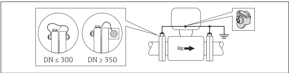
图 13 通过接地端子和管道法兰实现系统电势平衡
