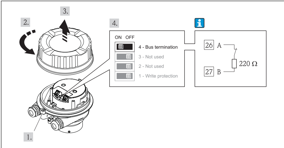
17 Abschlusswiderstand über DIP-Schalter auf Hauptelektronikmodul aktivierbar
