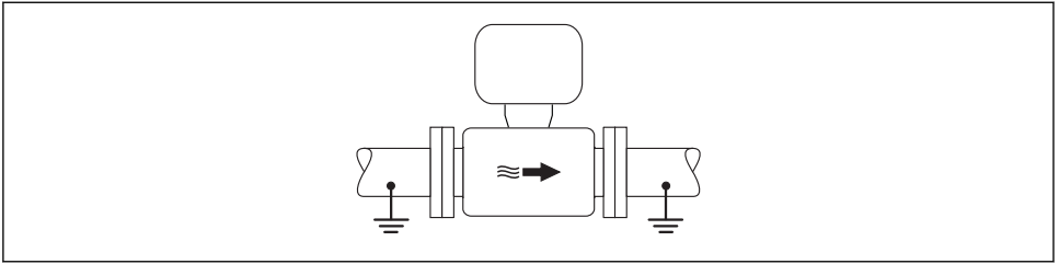
12 Potenzialausgleich über Messrohr
