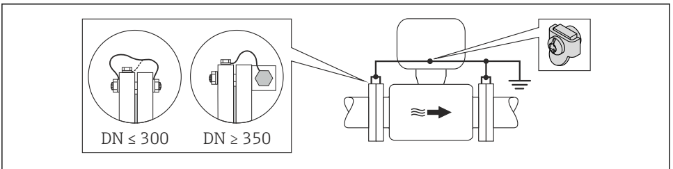
13 Potenzialausgleich über Erdungsklemme und Rohrleitungsflansche
