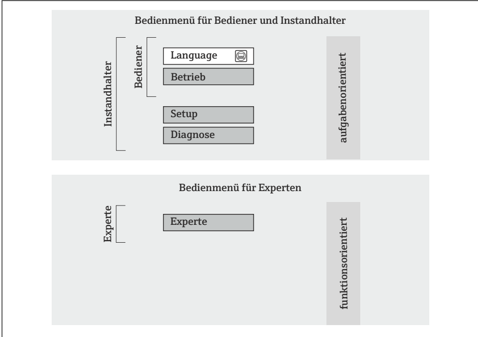
18 Schematischer Aufbau des Bedienmenüs
