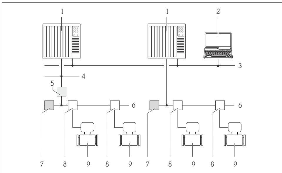
13 Possibilités de configuration à distance via réseau FOUNDATION Fieldbus
