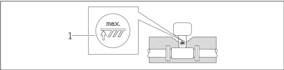
1 Altura máxima del aislante
