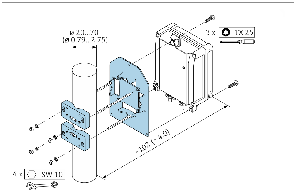
14 单位: mm (in)
