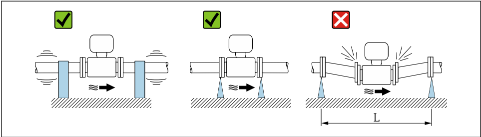
图 6 仪表防振措施 ( L > 10 \text{ m} (33 ft))
