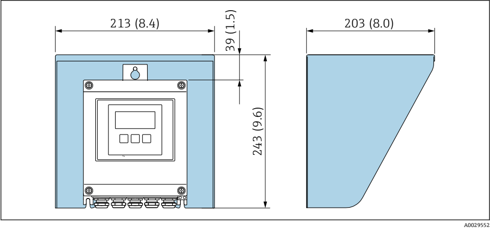
4 Proline 500 (数字式)的防护罩
