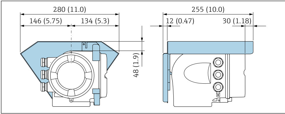
图 5 Proline 500 的防护罩
