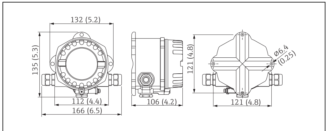
Abmessungen des Feldanzeigers, Maßeinheit mm (in)
