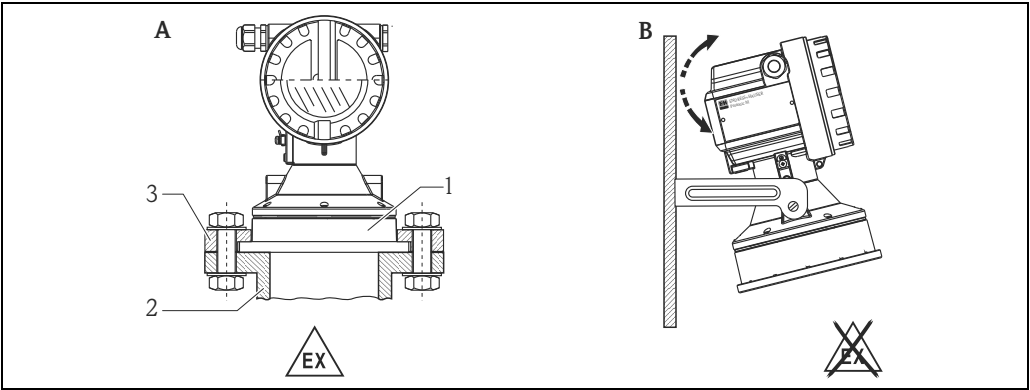
A Montage mit Überwurfflansch (z.B. Ex-Bereich, Zone 20) 1 Sensor, 2 Stützen, 3 Überwurfflansch B Montage mit Montagebügel (Nicht-Ex-Bereich, Zone 20)
