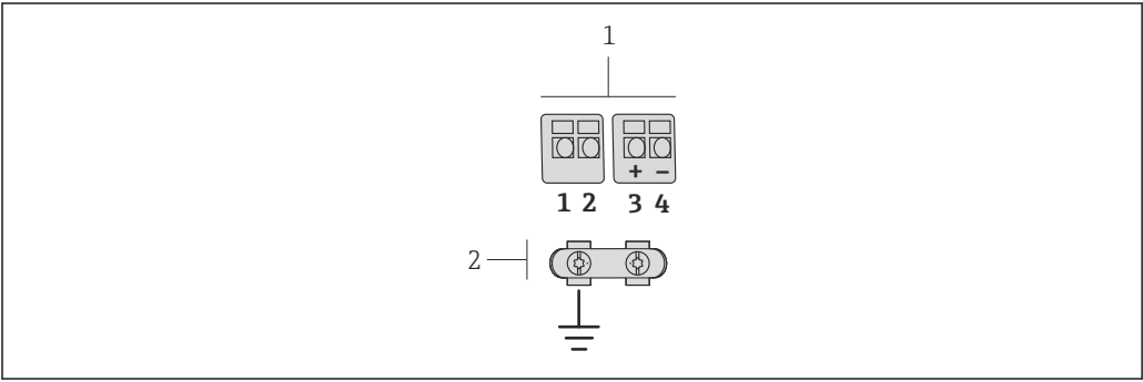
10 Bornes de raccordement pour le compartiment de raccordement dans le support mural du transmetteur et le boîtier de raccordement du capteur
