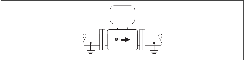
13 Potentialutjämning via mätörret
