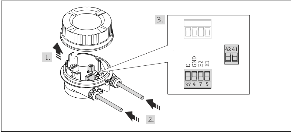
12 Sensor: anslutningsmodul
