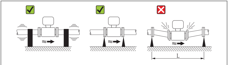
4 Mått för att undvika vibrationer ( L > 10\text{ m} (33 ft))
