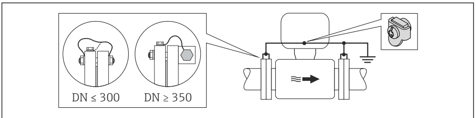
14 Potentialutjämning via jordanslutning och rörflänsar
